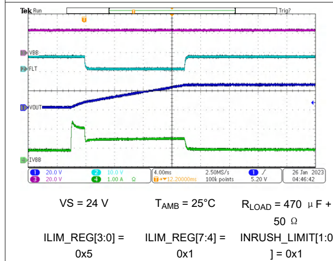
图 6-3. Charging a 470-µF Capacitor
