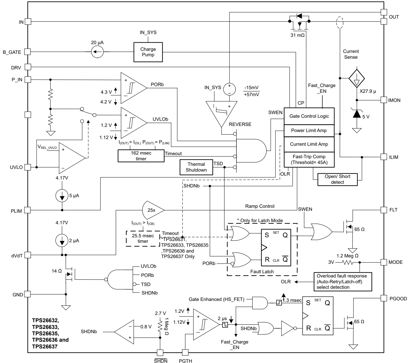
图 8-2. TPS26632, TPS26633, TPS26635, TPS26636 和 TPS26637 功能块图
