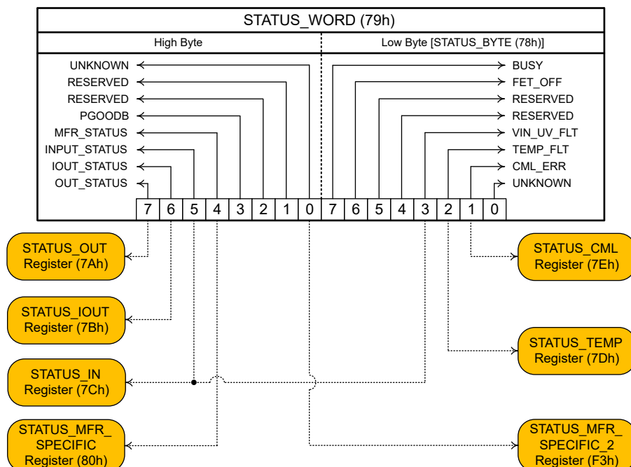
图 8-18. Status Register Bit Map
