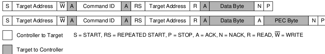
图 8-13. Read Byte
