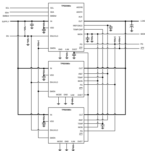
简化原理图
