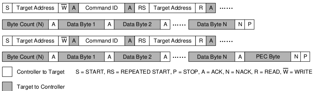
图 8-16. Block Read
