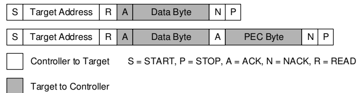
图 8-11. Receive Byte
