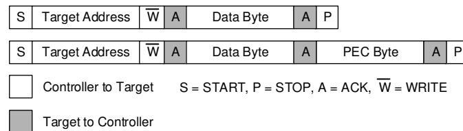
图 8-10. Send Byte
