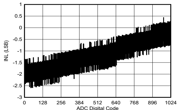
图 7-24. ADC INL
