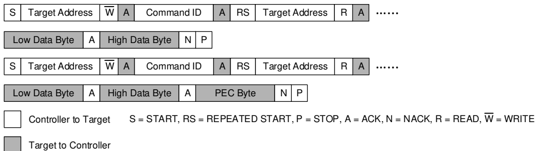
图 8-15. Read Word
