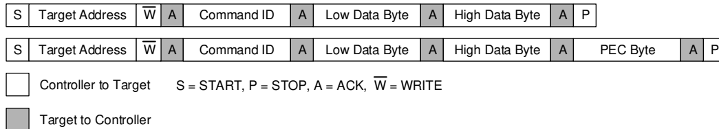
图 8-14. Write Word
