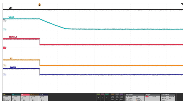
图 7-43. Power Down Using EN With Output Discharge
