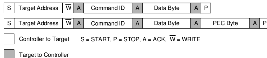
图 8-12. Write Byte
