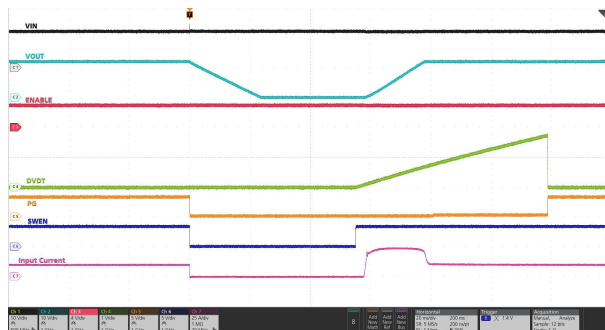
图 7-37. Power Down Using PMBus Command
