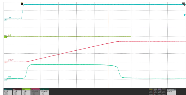
图 6-32. Input Hot-Plug
