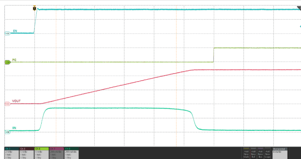
图 8-4. Power Up
