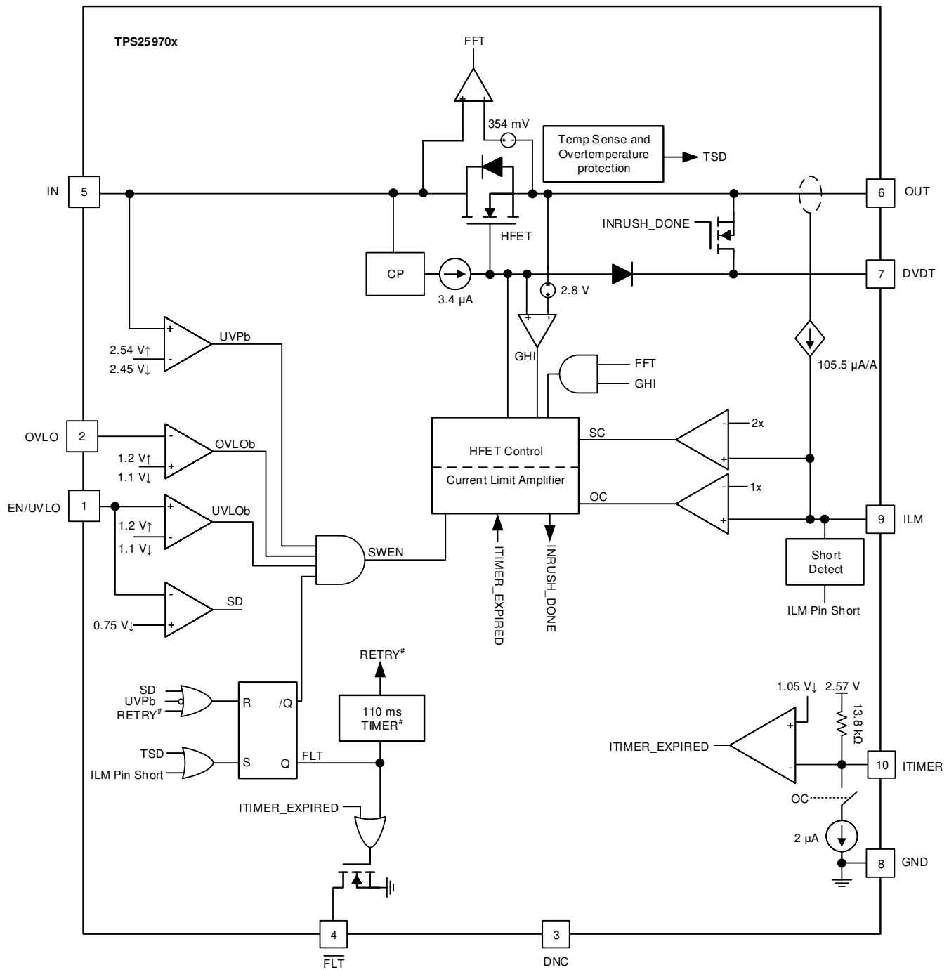
图 7-1. TPS25970x Block Diagram
