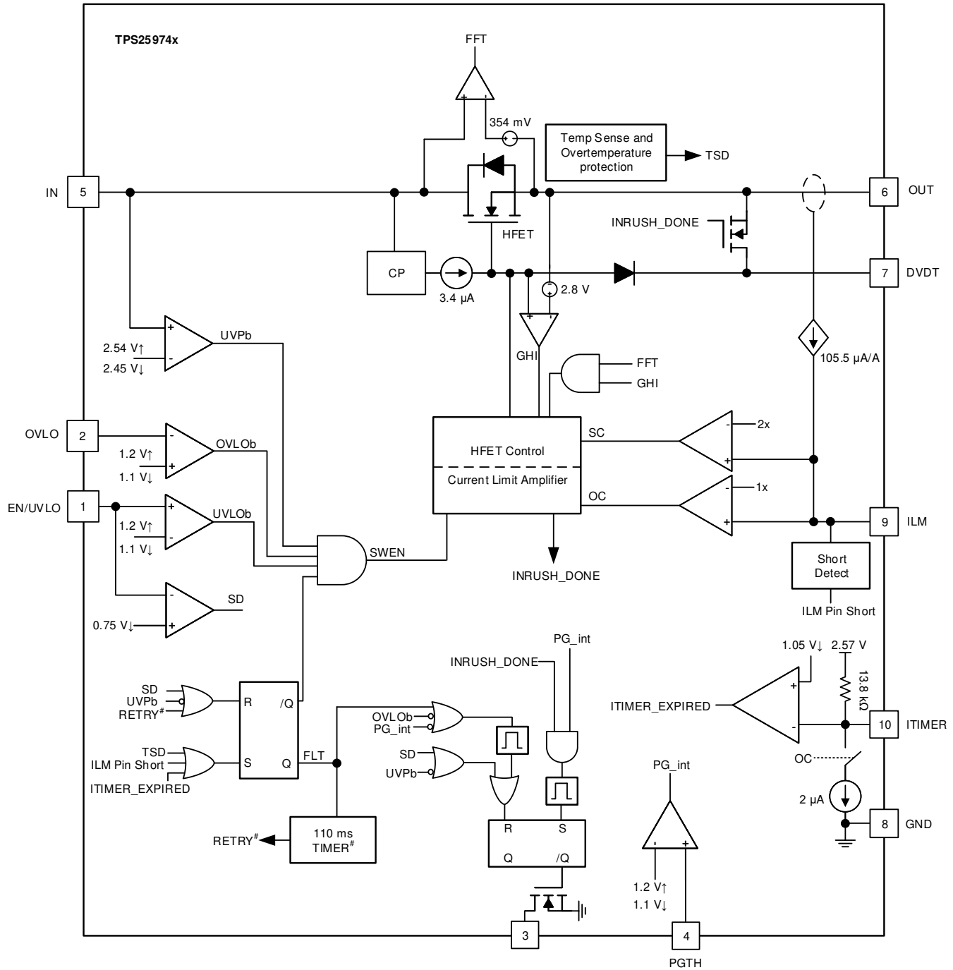
图 7-3. TPS25974x Block Diagram
