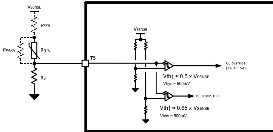
图 10-10. TS 输入
