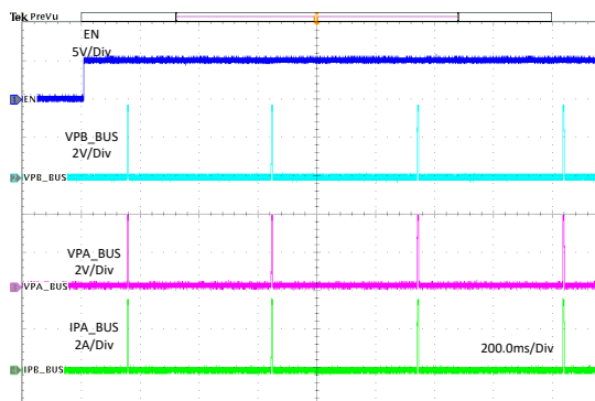
图 11-24. 启用至 1\Omega 负载
