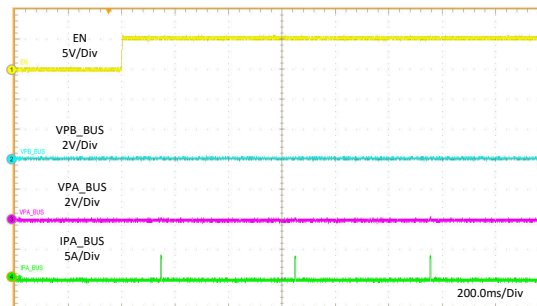
图 11-22. 启用至短接
