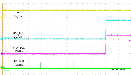
图 11-23. 短路恢复
