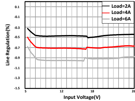
图 11-6. 线路调节
