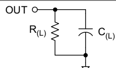
图 9-1. OUT 上升/下降测试负载图
