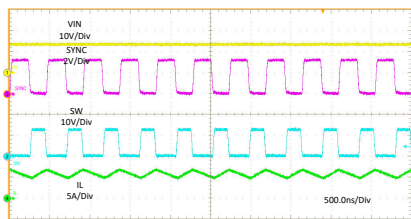
图 10-9. Synchronizing to External 2.2-MHz Clock
