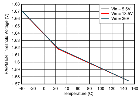
图 8-4. Precision USB PA/PB Enable Threshold
