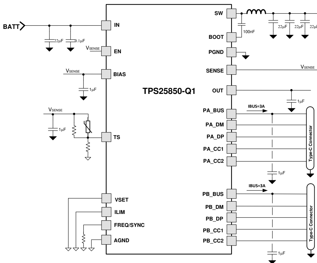
图 11-1. TPS25850-Q1 Typical Application Circuit for 2.1-MHz f_{sw}
