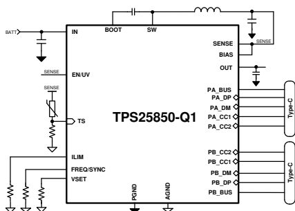
简化版原理图 TPS25850-Q1
