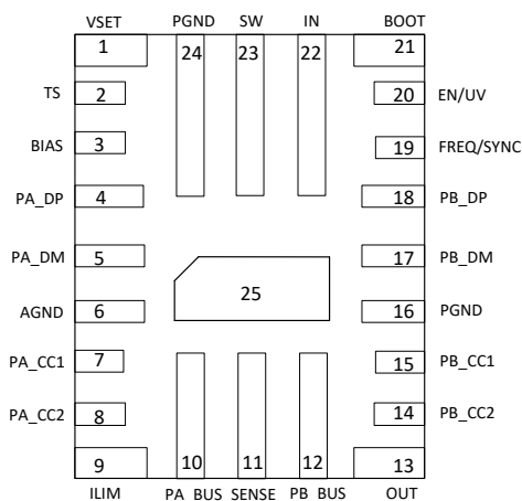
图 7-1. TPS25850-Q1 RPQ Package 25-Pin (QFN) Top View
