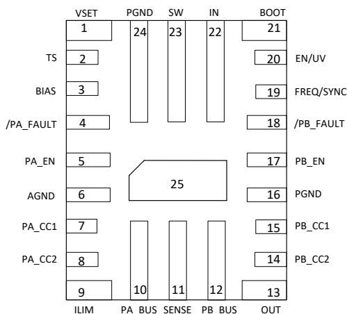
图 7-3. TPS25852-Q1 RPQ Package 25-Pin (QFN) Top View
