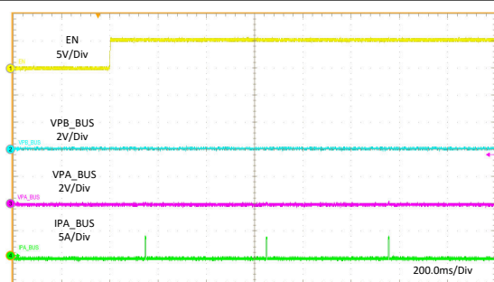
图 11-20. Rd Assert
