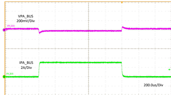
图 11-5. Load Regulation
