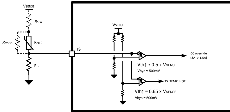
图 10-16. TS Input
