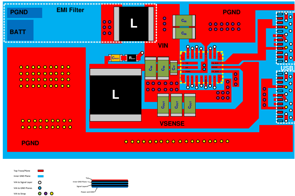
图 13-1. Layout Example
