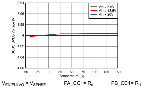
图 8-7. DCDC UVLO Threshold
