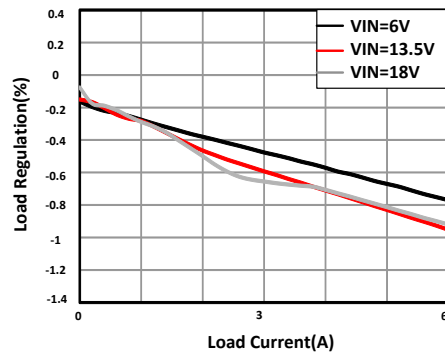
图 11-5. Load Regulation
