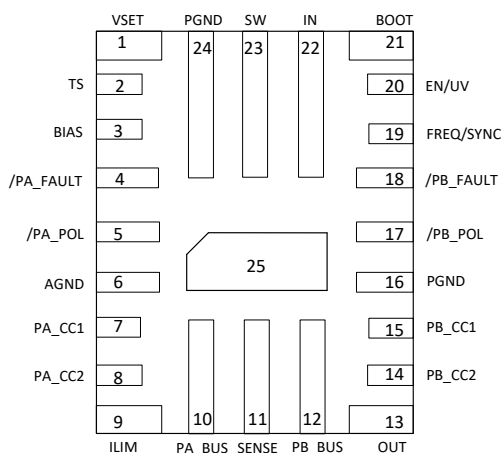
图 7-2. TPS25851-Q1 RPQ Package 25-Pin (QFN) Top View
