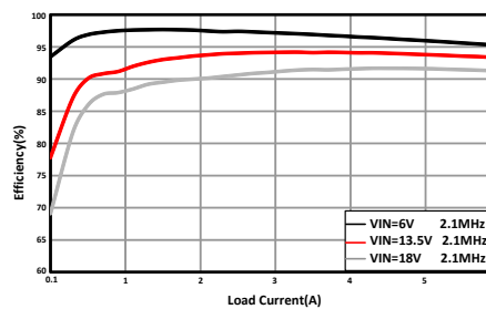
效率与输出电流间的关系
