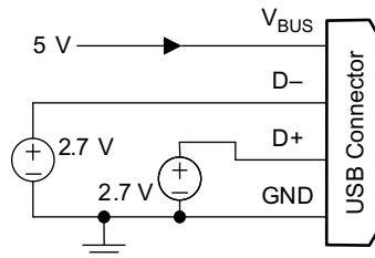
图 10-22. Divider 3 Mode
