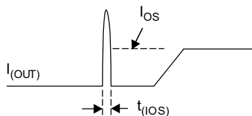
图 9-1. Short-Circuit Parameters
