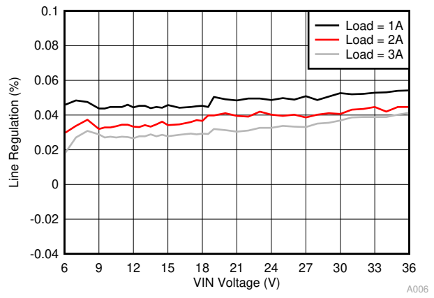
图 11-7. Line Regulation
