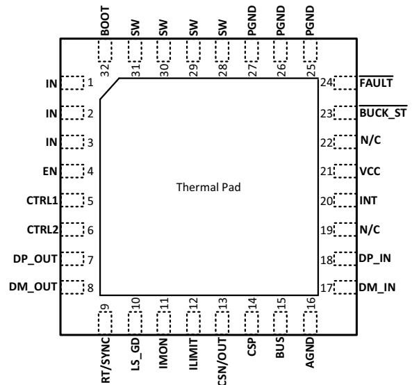
图 7-2. TPS25840QWRHBRQ1, TPS25842QWRHBRQ1 Package 32-Pin (VQFN) Top View (2)
