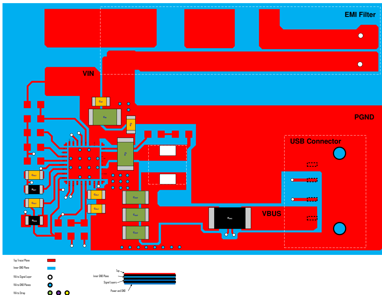
图 13-1. Layout Example
