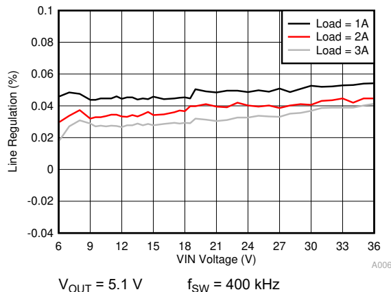
图 11-7. Line Regulation
