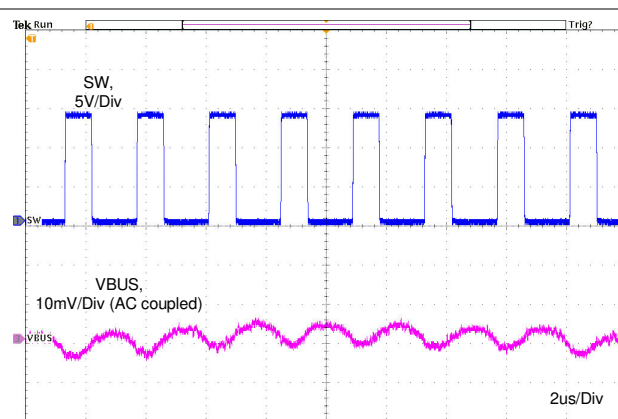
图 11-15. No Load Output Ripple
