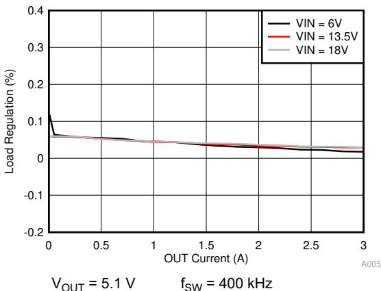
图 11-6. Load Regulation
