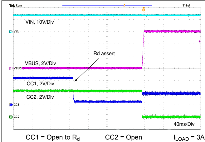
图 11-20. Rd Assert
