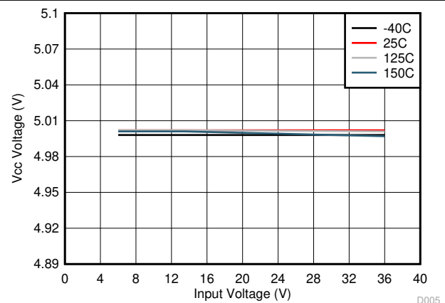
图 8-6. VCC vs Input Voltage
