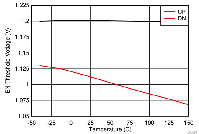
图 8-4. Precision Enable Threshold
