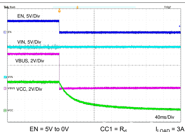
图 11-19. Shutdown Relate to EN
