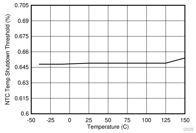
图 8-28. NTC Temperature Shutdown Threshold (TPS25833-Q1)
