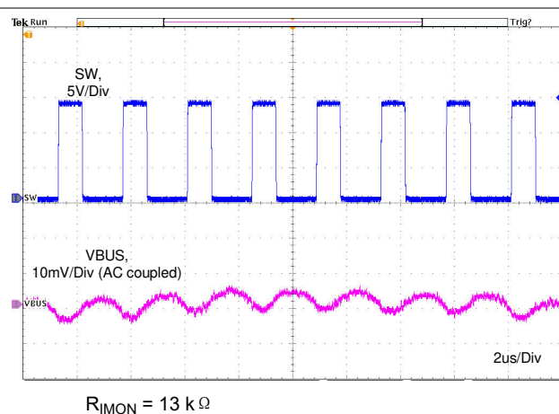
图 11-15. No Load Output Ripple
