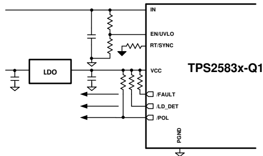
图 10-14. V_{\text{CONN}} Source Using External LDO
