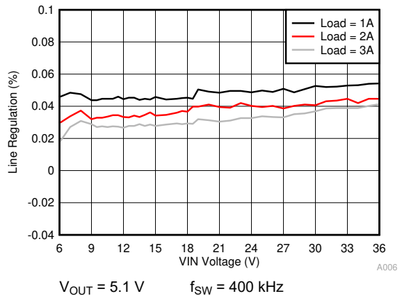
图 11-7. Line Regulation
