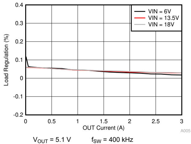
图 11-6. Load Regulation
