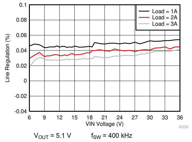
图 11-7. Line Regulation
