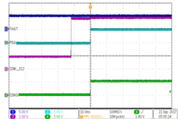
图 14. Sink Detach Event
