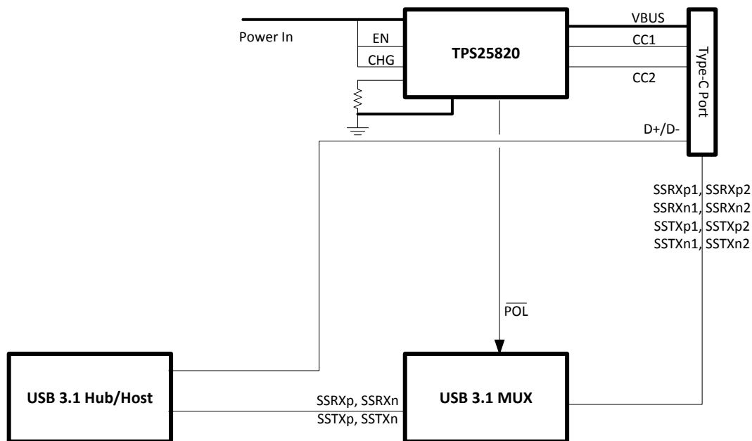
图 20. USB 3.1 Type-C Charging Port
