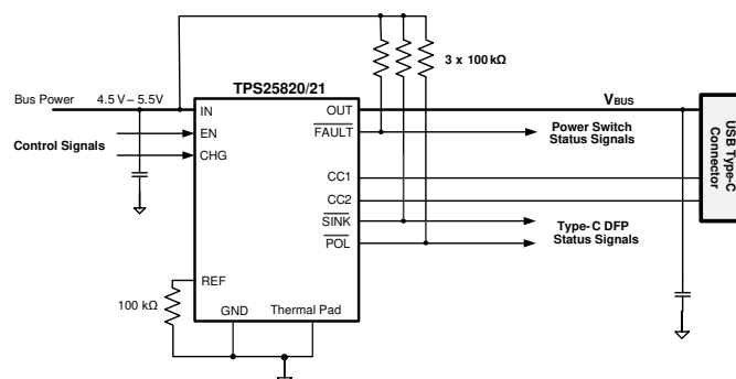
简化原理图
