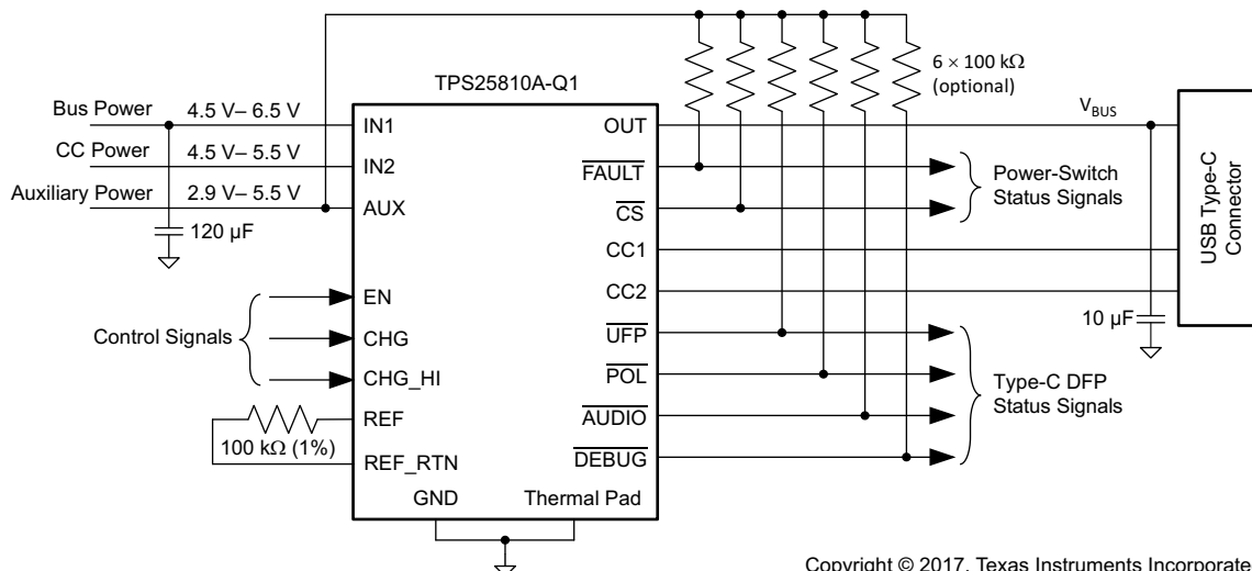
简化原理图
