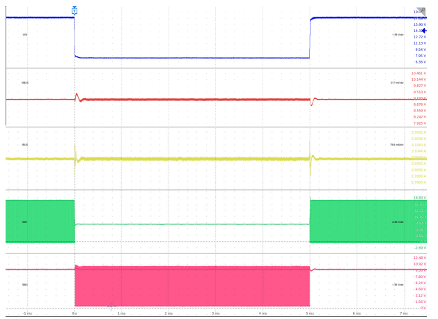
图 10-37. Line Transient: V_{BUS} = 9\text{ V}
