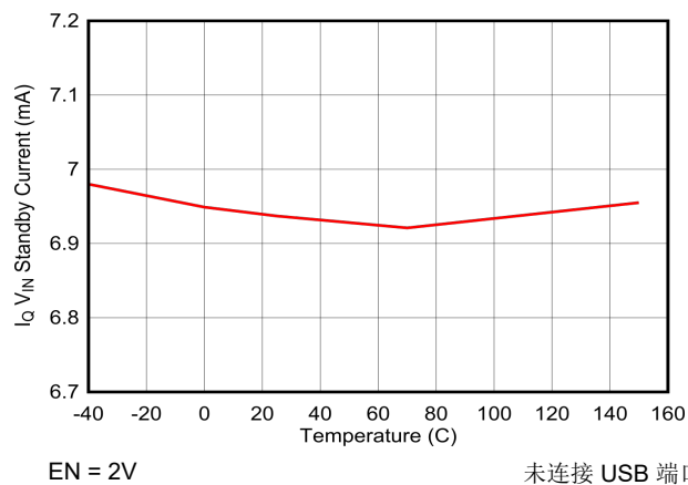
图 6-2. I_Q V_{IN} 待机电流与温度间的关系
