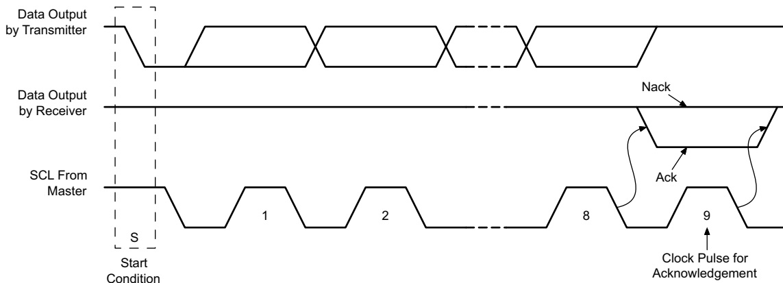
图 8-38. I 2 C 确认
