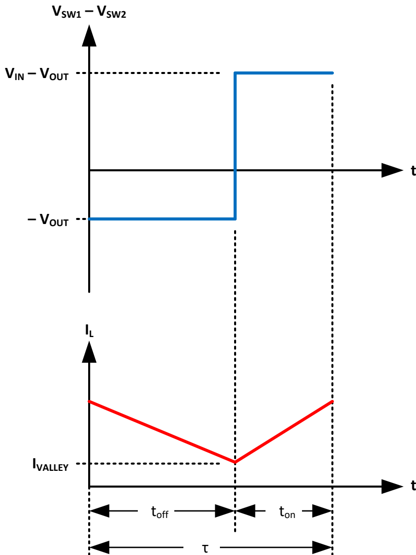
图 8-9. 降压状态
