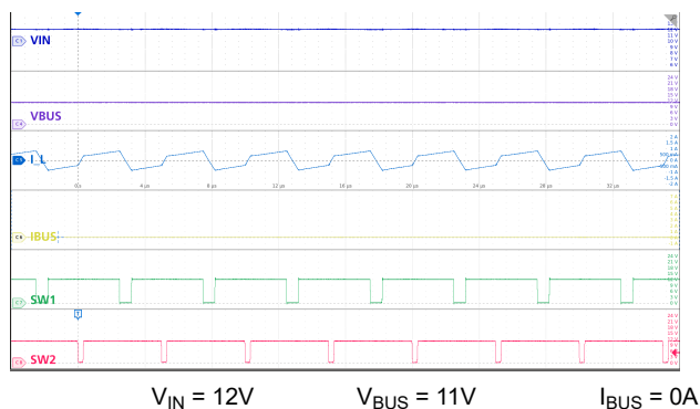
图 9-23. 降压/升压模式： V_{IN} \neq V_{BUS} ，空载
