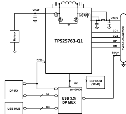
TPS25763-Q1 简化原理图
