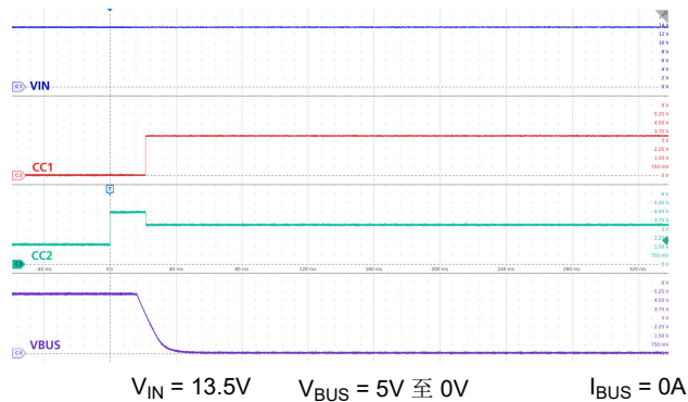
图 9-13. Type-C 断开
