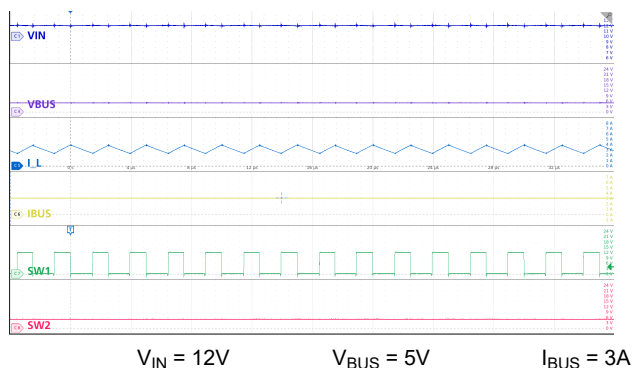
图 9-20. 降压模式：标称 V_{IN} ，3A 负载
