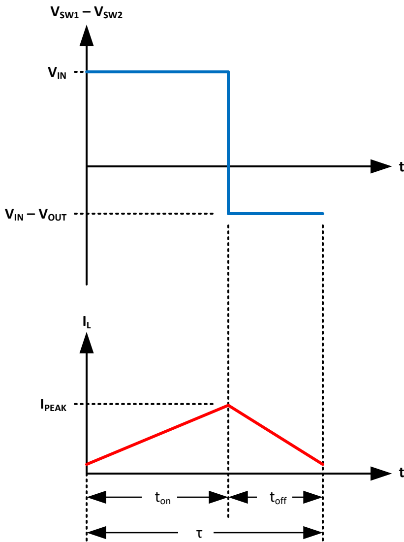
图 8-12. 升压状态
