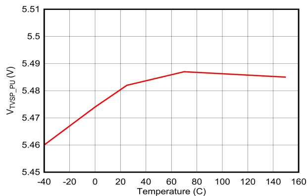
图 6-14. V_{TVSP\_PU} 与温度间的关系
