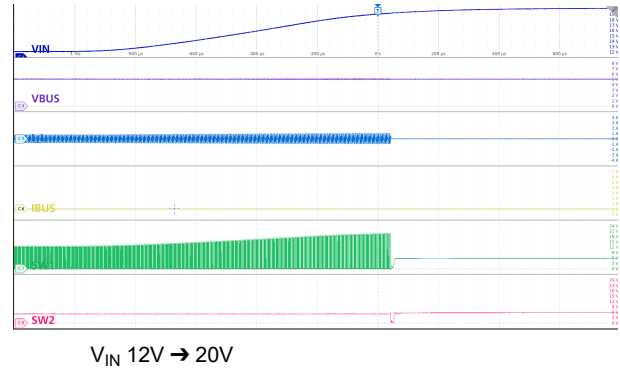
图 9-27. V_{IN(OVP)} 进入
