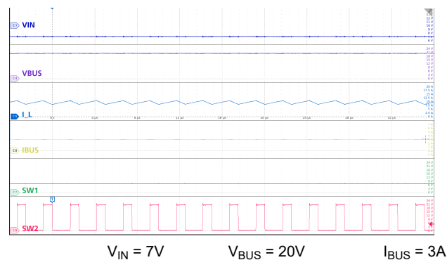
图 9-16. 升压模式：低 V_{IN} ，3A 负载
