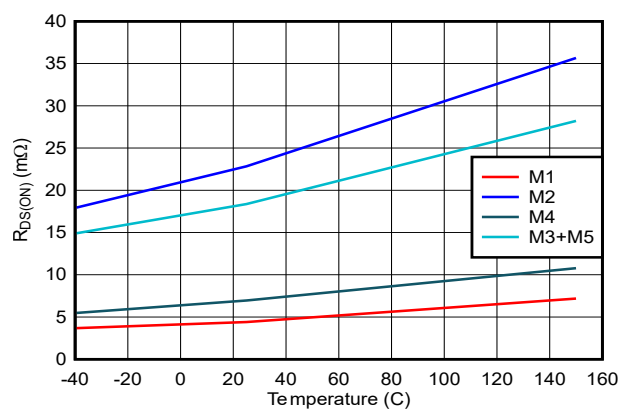
图 6-16. 降压/升压功率 FET R_{DS(on)} 与温度间的关系
