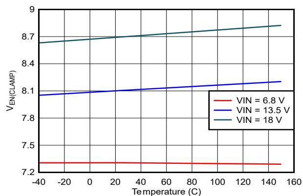
图 6-4. EN 钳位电压与温度间的关系
