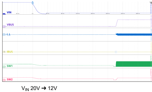
图 9-28. V_{IN(OVP)} 恢复
