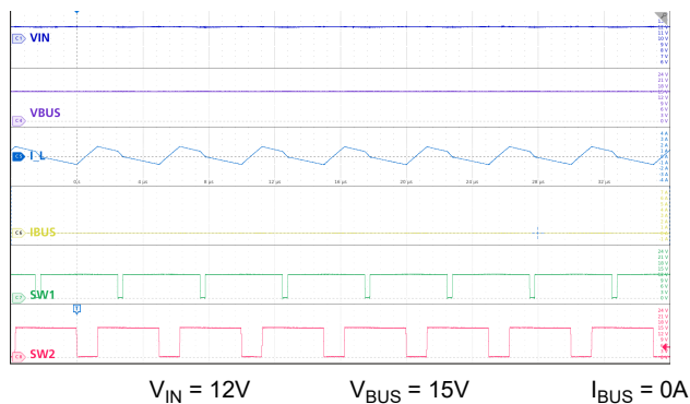
图 9-25. 降压/升压模式：标称 V_{IN} ，空载
