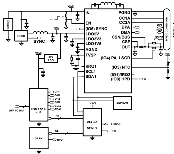
图 9-1. 具有 DisplayPort 交替模式并通过 I2C 实现多路复用器控制的简化版单端口 PD 充电器
