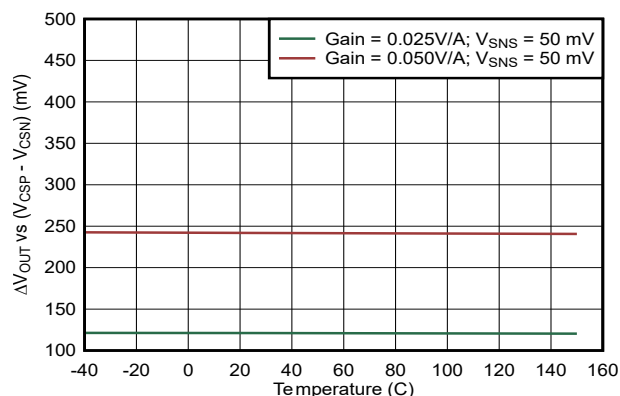
图 6-30. 电缆压降补偿与温度间的关系
