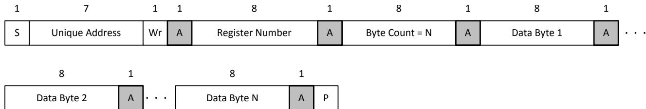
图 8-39. I 2 C 唯一地址写入寄存器协议
