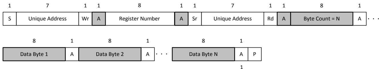
图 8-40. I 2 C 唯一地址读取寄存器协议
