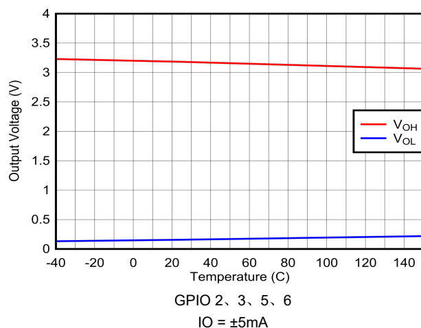
图 6-45. GPIO : 输出电压与输出电流和温度间的关系
