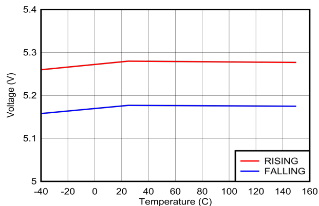
图 6-6. V_{IN(UVLO)} 与温度间的关系
