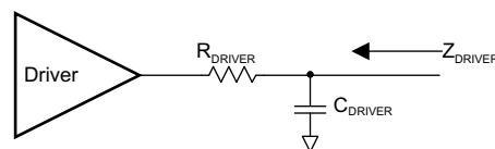
图 8-25. ZDRIVER 电路
