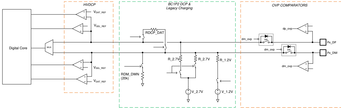
图 8-33. BC1P2 功能框图
