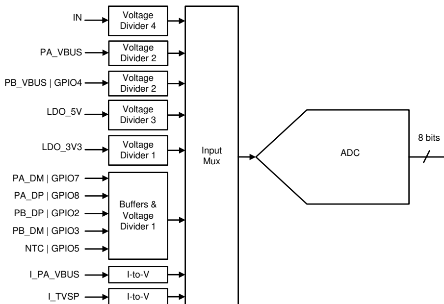
图 8-31. SAR ADC
