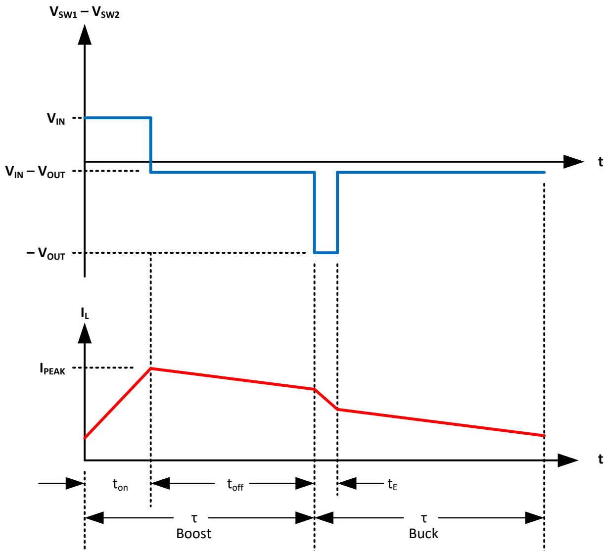
图 8-11. 升压转换
