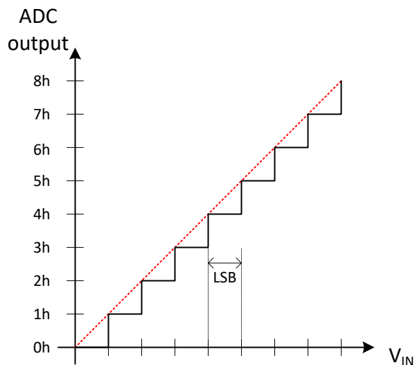
图 8-32. ADC 转换
