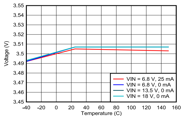
图 6-10. LDO_3V3 与 V_{IN} 和温度间的关系
