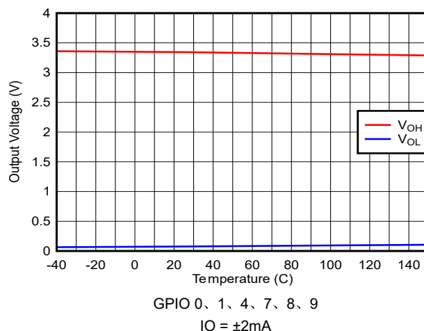
图 6-44. GPIO : 输出电压与输出电流和温度间的关系
