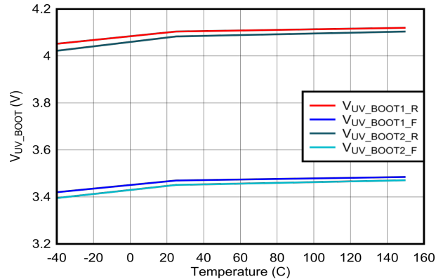
图 6-22. BOOTx UVLO 与温度间的关系
