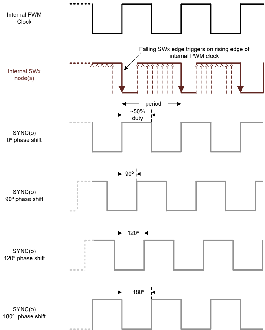
图 8-15. SYNC(o) 相移
