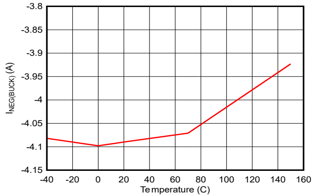
图 6-21. 降压负电流限制与温度间的关系
