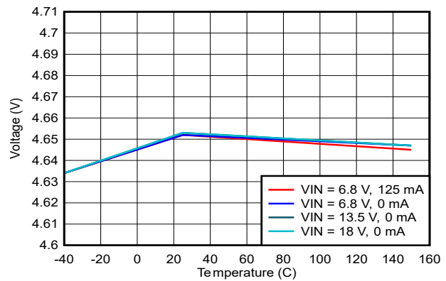
图 6-8. LDO_5V 与 V_{IN} 和温度间的关系
