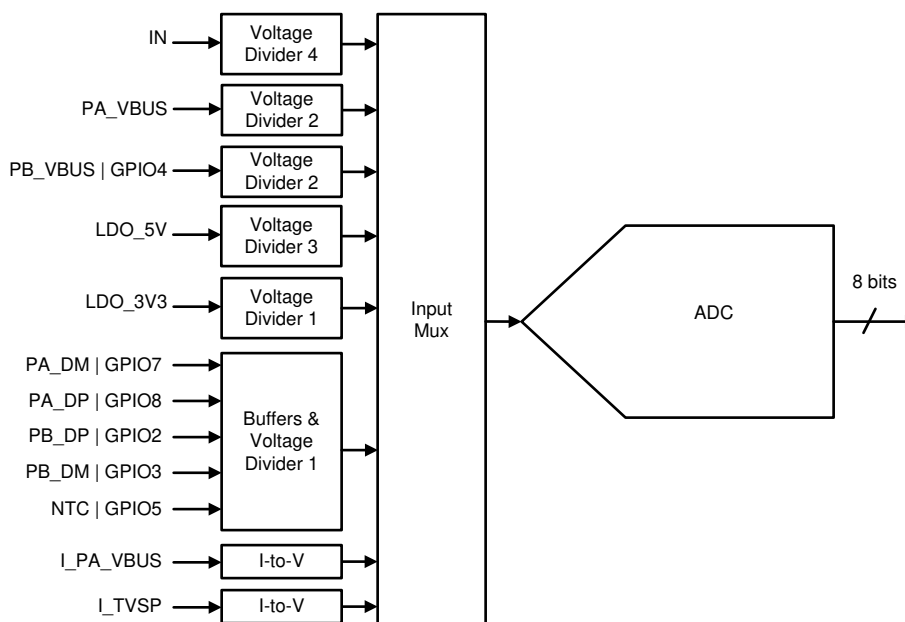
图 8-30. SAR ADC
