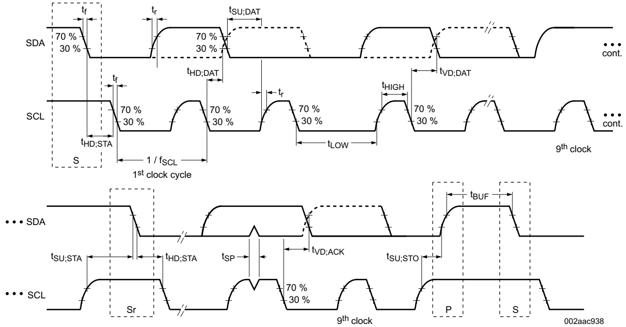
图 7-1. I²C 目标接口时序
