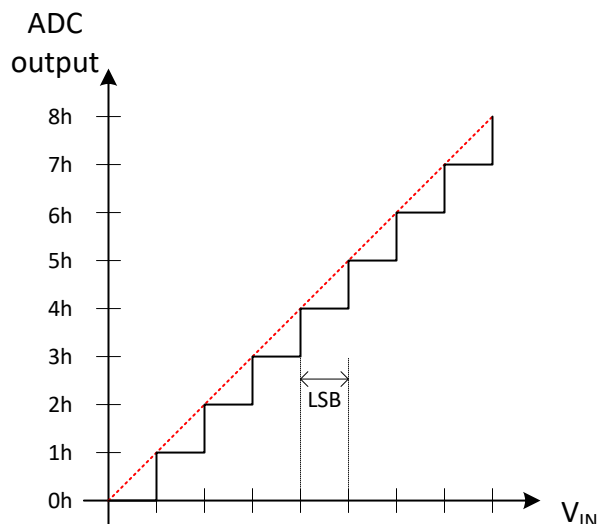
图 8-31. ADC 转换
