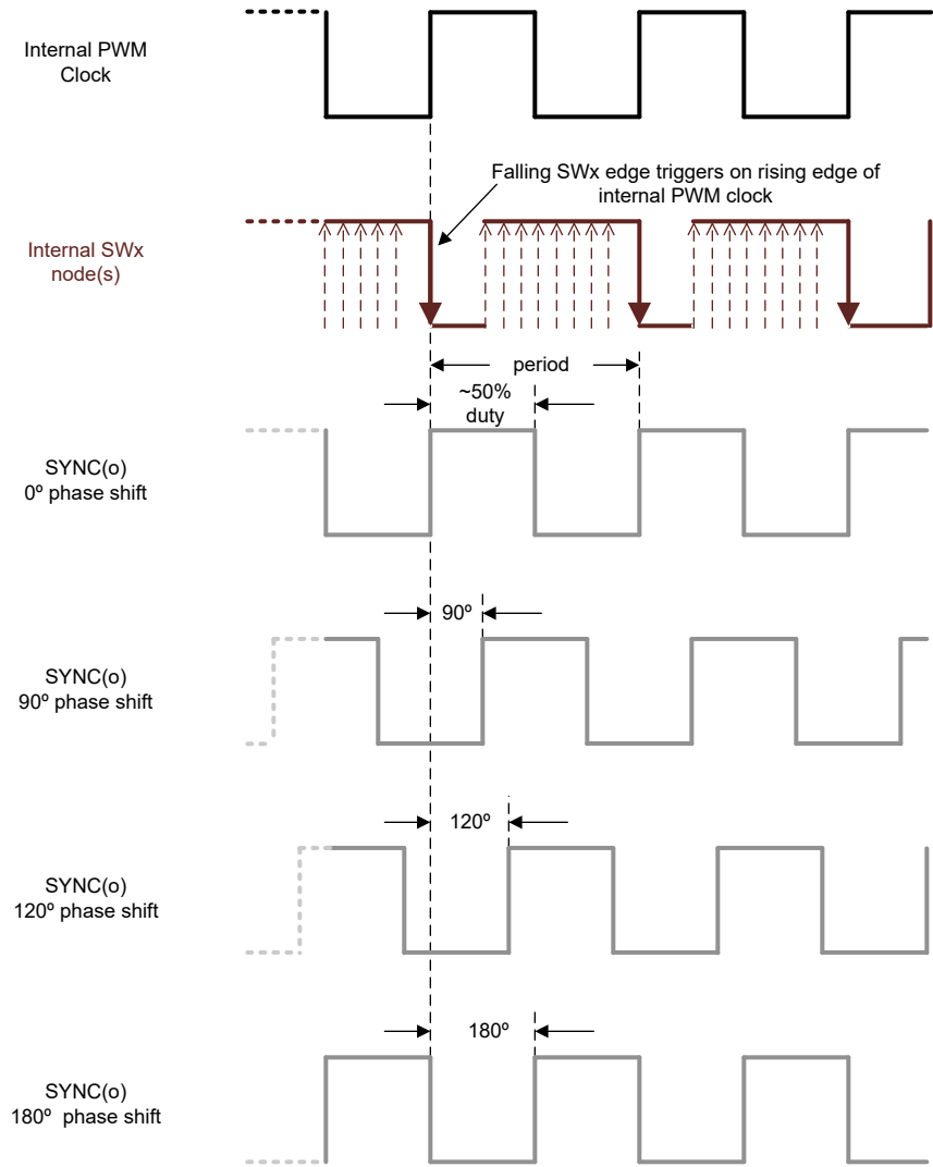
图 8-14. SYNC(o) 相移
