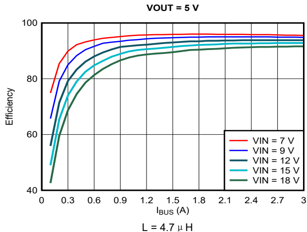
图 9-6. 效率与输出电流 ( I_{OUT} ) 间的关系, V_{OUT} = 5V
