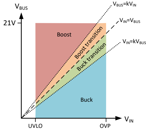
图 8-12. 工作区域
