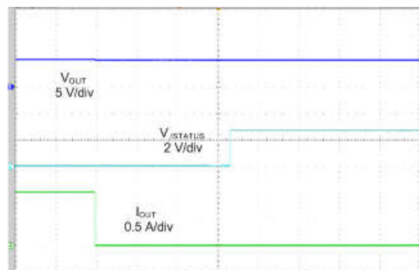
图 6-24. Hot Short
