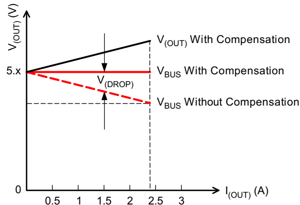
图 8-1. Voltage Drop
