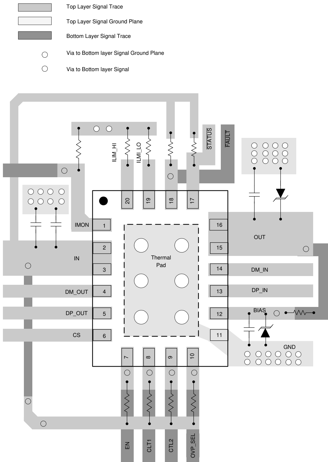
图 11-1. TPS254900A-Q1 Layout Diagram
