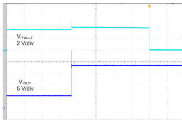
图 6-25. Load-Detection Set Time
