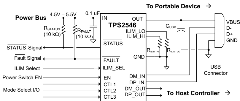
简化电路原理图
