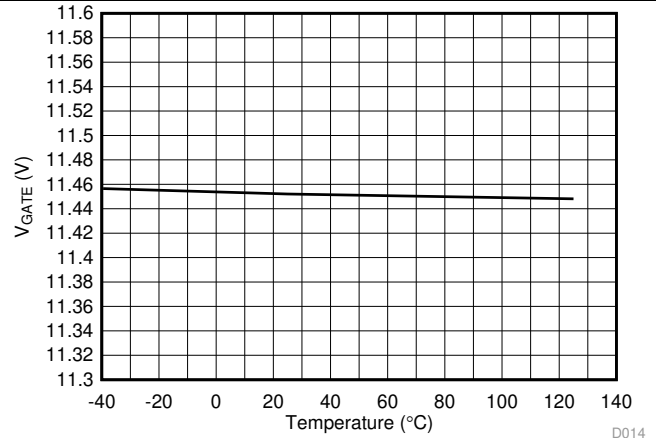
图 14. 栅极电压 (端口开启) 与温度间的关系
