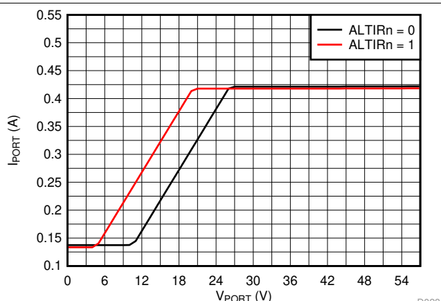
图 26. 浪涌电流折返与端口电压间的关系
