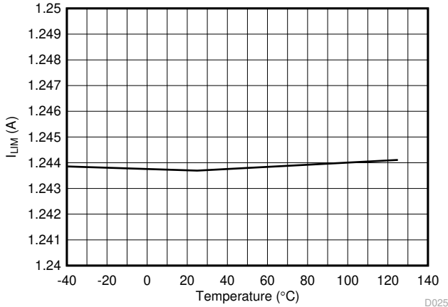
图 6-25. 2x 模式 ( 2\text{xFBn} = 1 ) 电流限制与温度间的关系
