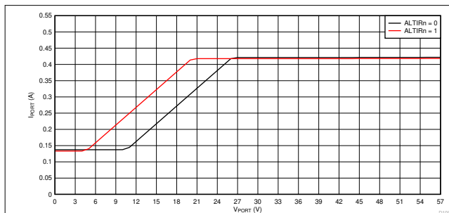
图 8-2. 浪涌期间折返 (端口开启时) : I_{LIM} 与 V_{port} 间的关系
