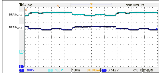
图 9-12. 4 线对低电阻 (11k \Omega ) 检测特征
