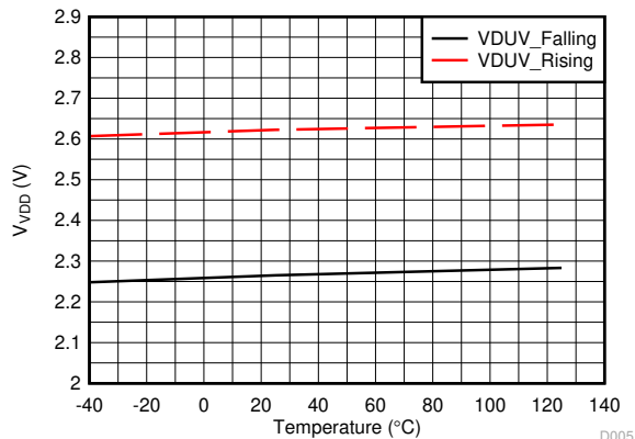
图 6-5. VDUV 阈值与温度间的关系
