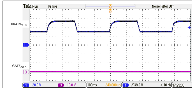
图 9-10. 2 线对开路检测特征
