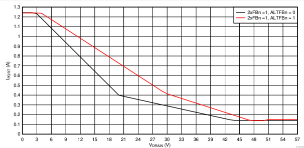
图 8-57. 2x 模式 (2xFBn = 1) 折返曲线， I_{PORT} 与 V_{DRAIN} 间的关系
