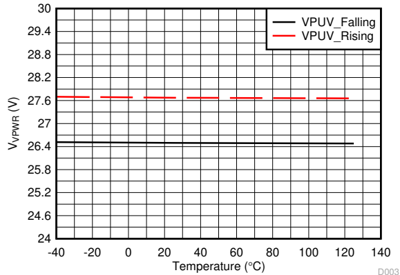
图 6-3. VPUV 阈值与温度间的关系
