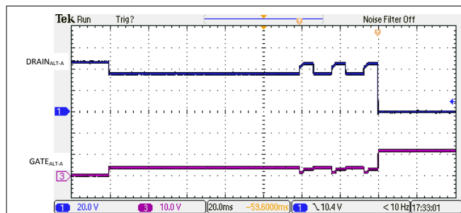
图 9-16. 2 线对 3 级侦测分类和开启
