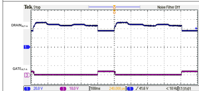
图 9-14. 具有有效 0-3 类负载的 2 线对半自动模式发现
