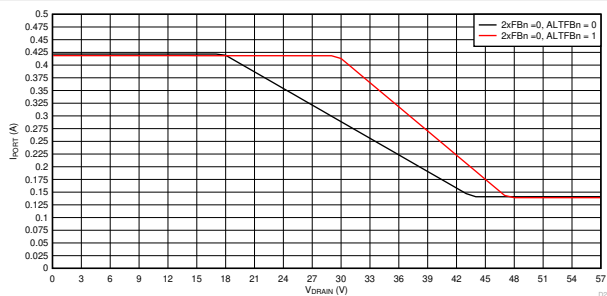
图 8-56. 1x 模式 (2xFBn = 0) 折返曲线， I_{PORT} 与 V_{DRAIN} 间的关系
