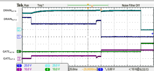
图 9-19. 4 线对单一特征 1 级侦测分级和开启
