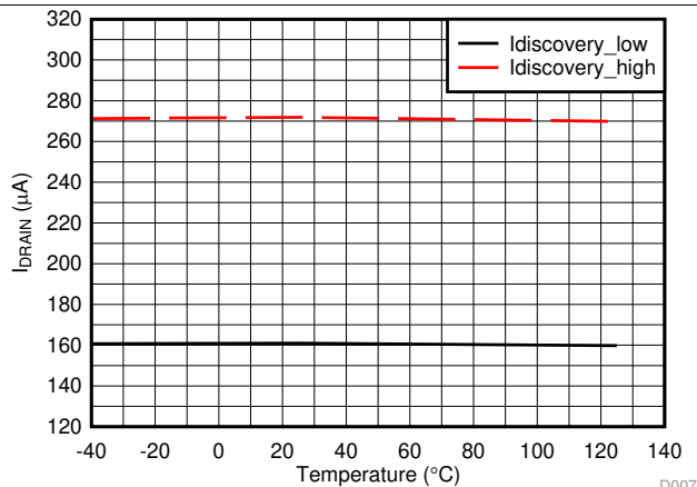
图 7. 发现电流与温度间的关系
