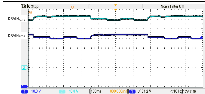
图 133. 4 线对低电阻 (11kΩ) 检测特征
