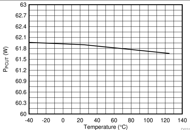
图 21. 4 线对 PCut 阈值 (60W) 与温度间的关系
