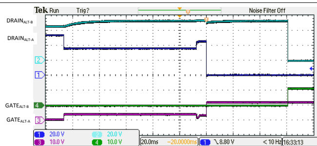
图 140. 4 线对单一特征 1 指分级和开启
