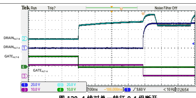
图 130. 4 线对单一-特征 0-4 级断开
