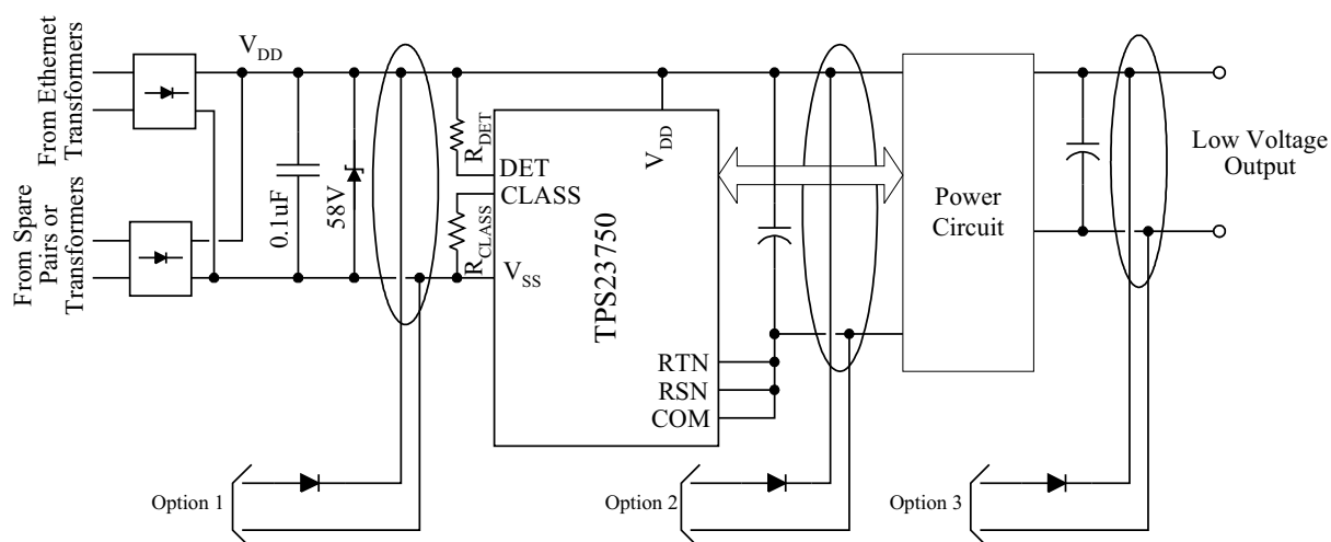
Figure 37. 辅助电源 ORing
