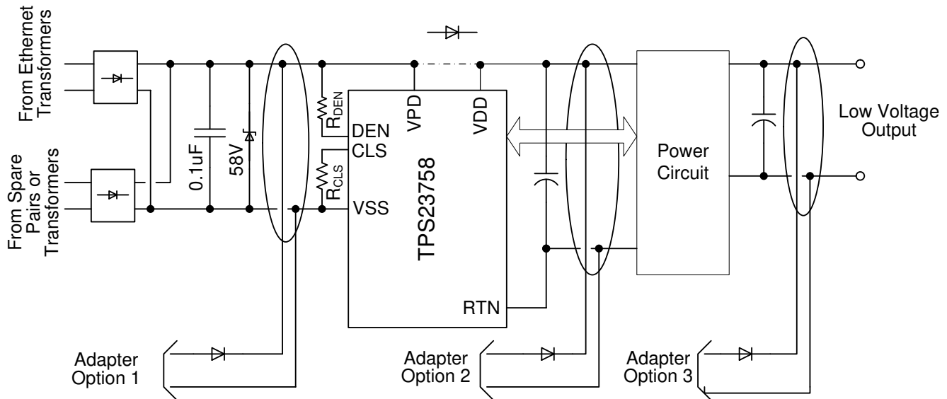
图 7-10. ORing Configurations
