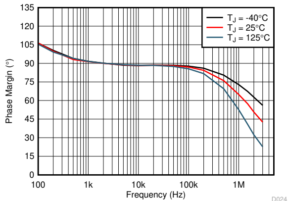
图 6-21. Error Amplifier Phase vs Frequency
