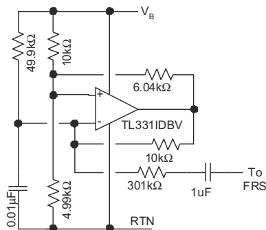
图 8-11. Frequency Dithering
