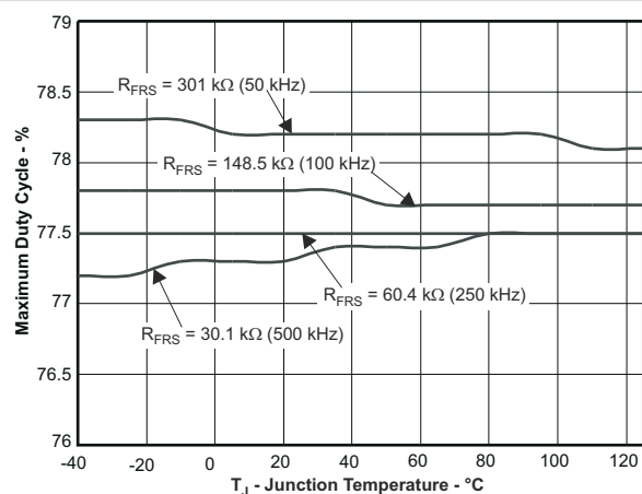
图 7-9. Maximum Duty Cycle vs Temperature
