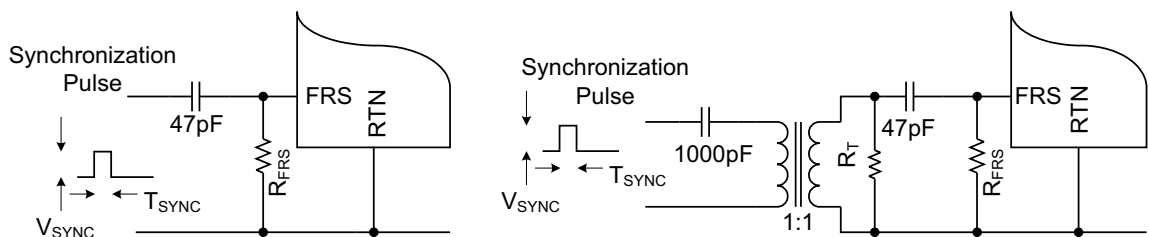
图 8-7. Synchronization
