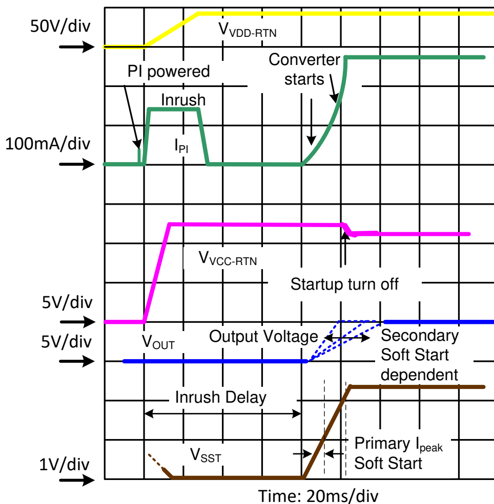
图 8-10. 加电和启动 - 具有光耦合器反馈
