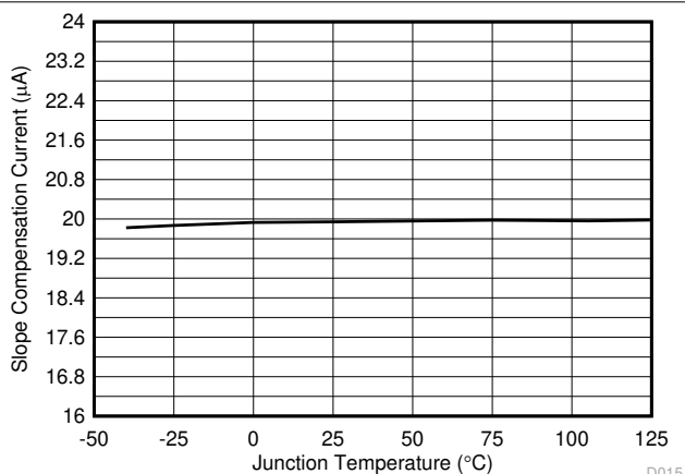
图 7-15. 斜坡补偿电流与温度间的关系
