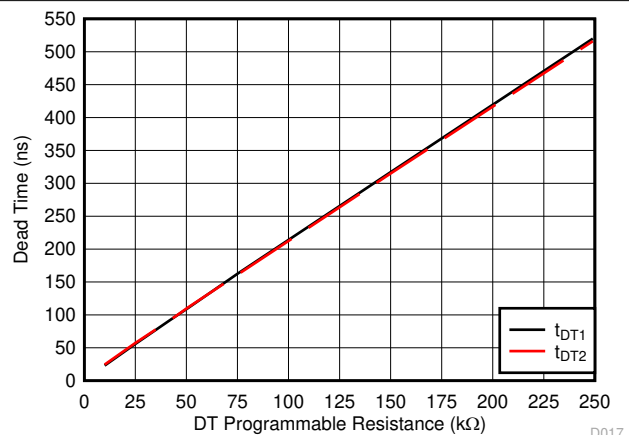
图 7-17. 死区时间与死区时间电阻 ( R_{DT} ) 间的关系
