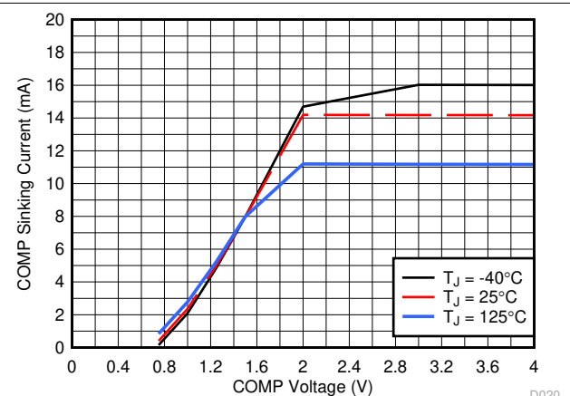
图 7-19. 误差放大器灌电流
