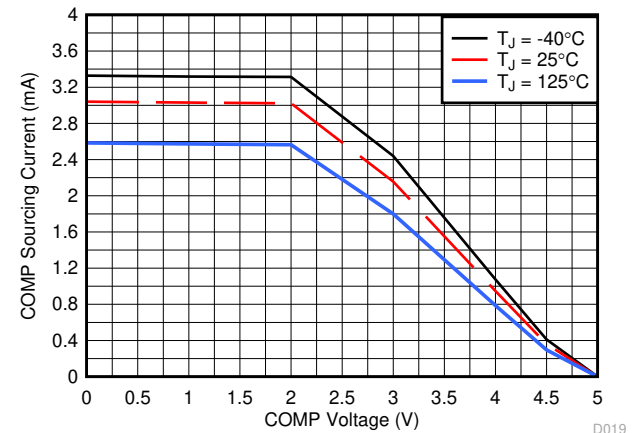
图 7-16. 误差放大器拉电流
