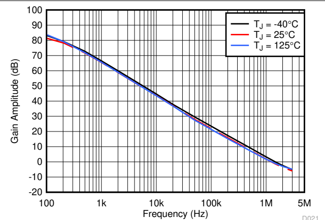
图 7-18. 误差放大器增益与频率间的关系
