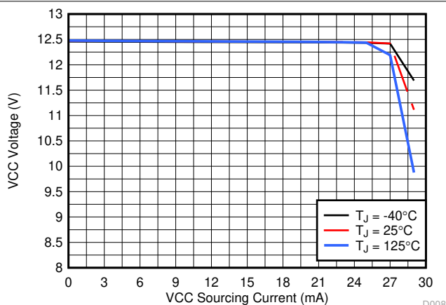
图 7-7. 转换器启动电压与电流间的关系
