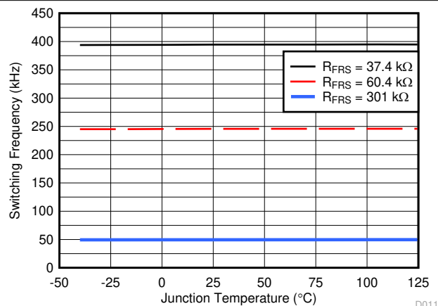
图 7-10. 开关频率与温度间的关系
