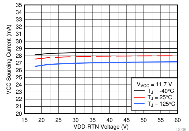
图 7-5. 转换器启动电流与 VDD 输入电压间的关系
