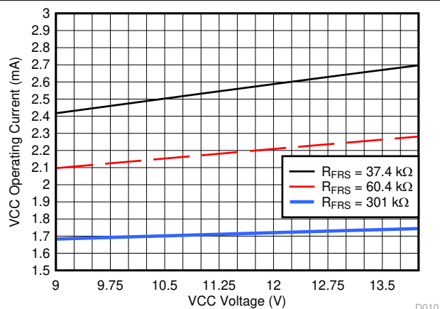
图 7-9. 控制器偏置电流与电压间的关系
