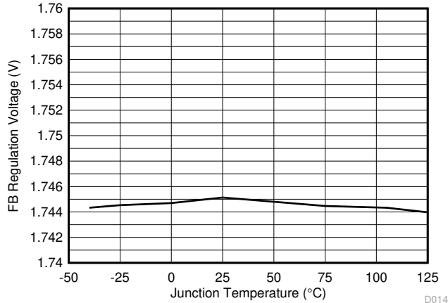
图 7-13. 反馈调节电压与温度间的关系
