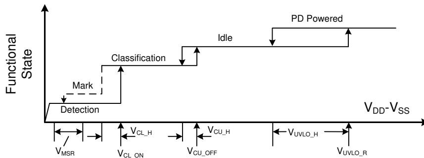
图 8-6. 阈值电压
