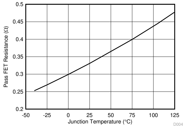
图 7-3. 导通 FET 电阻与温度间的关系
