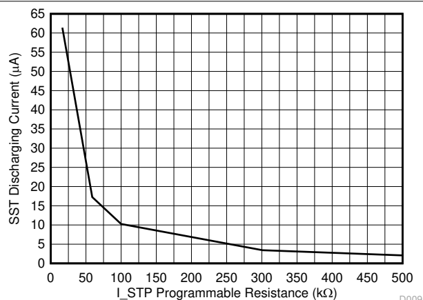
图 7-8. 控制器 SST 软停止灌电流与已变成电阻间的关系
