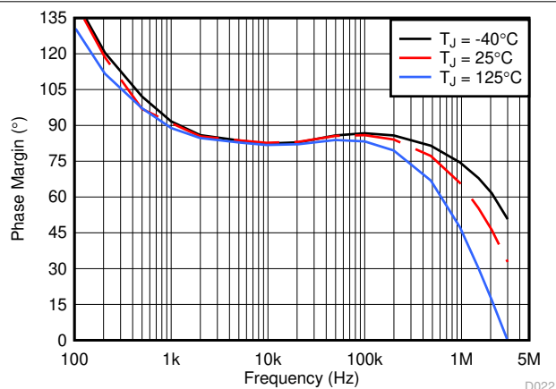
图 7-19. 误差放大器相位与频率间的关系
