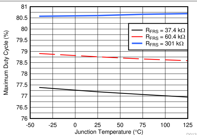
图 7-12. 最大占空比与温度间的关系
