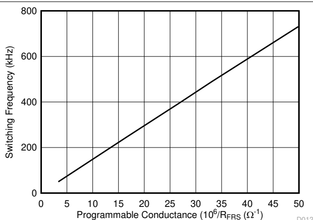
图 7-11. 开关频率与已编程电阻间的关系
