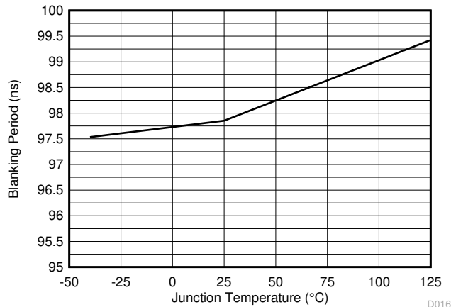
图 7-15. 消隐周期与温度间的关系
