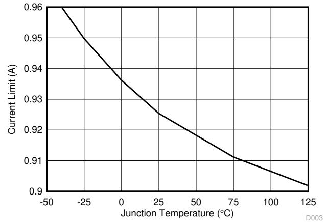
图 7-2. PoE 电流限制与温度间的关系
