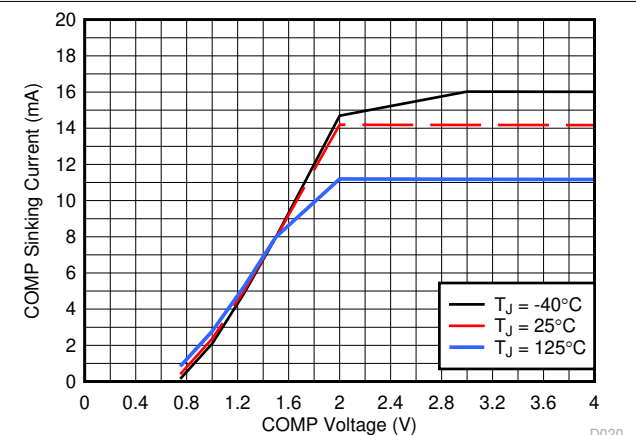
图 7-17. 误差放大器灌电流
