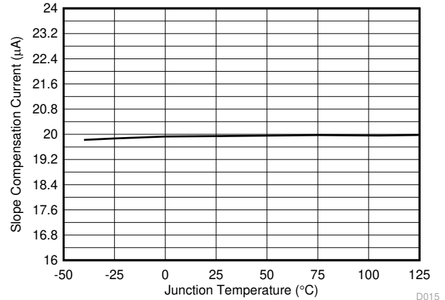
图 7-14. 斜坡补偿电流与温度间的关系
