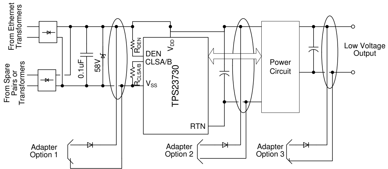
图 8-15. ORing 配置
