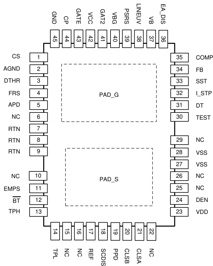
图 6-1. RMT 封装 45 引脚 VQFN 俯视图
