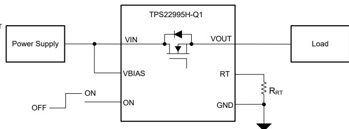
典型应用图
