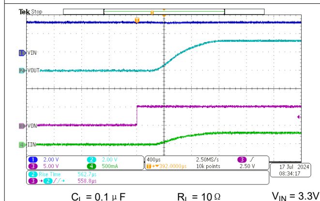
图 10-4. TPS22991C 的典型导通
