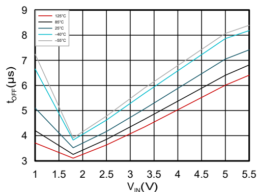
图 7-8. 关断时间与输入电压间的关系
