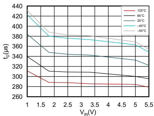
图 7-13. 延迟时间与输入电压间的关系
