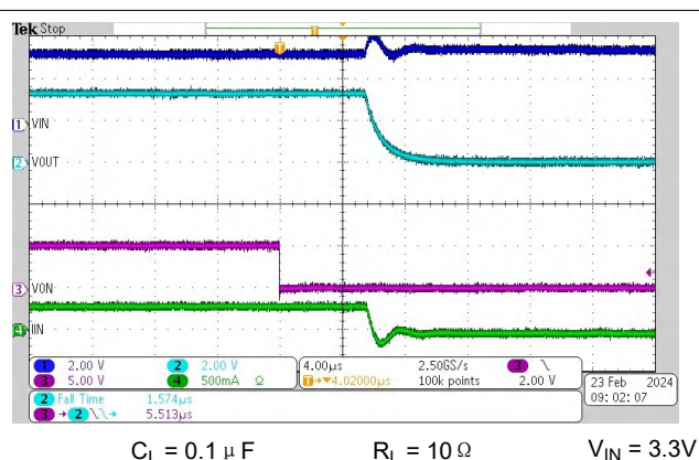
图 10-3. TPS22991B 的典型关断
