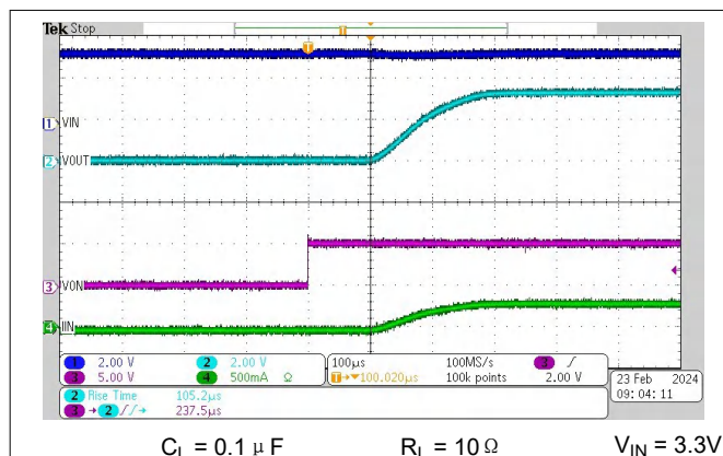
图 10-2. TPS22991B 的典型导通
