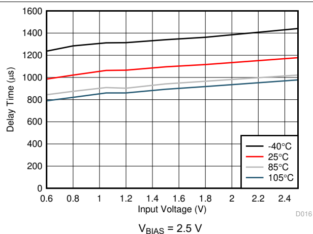
图 6-19. Delay Time vs Input Voltage
