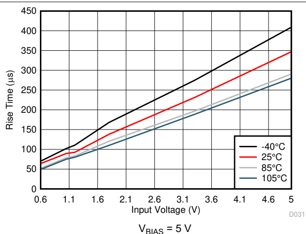
图 6-44. Rise Time vs Input Voltage
