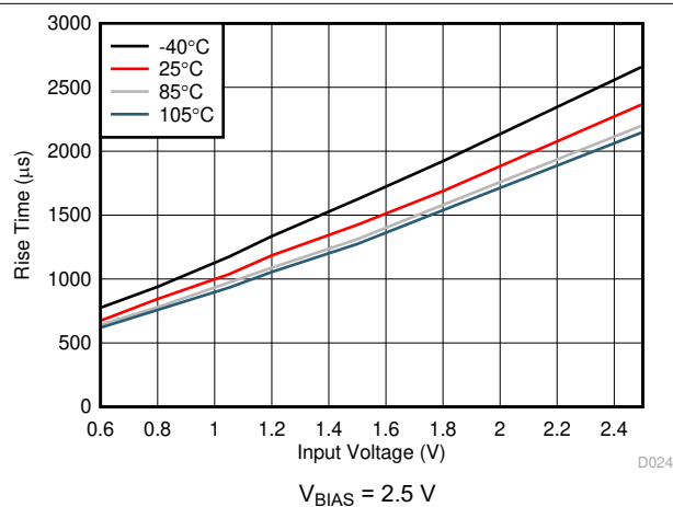
图 6-29. Rise Time vs Input Voltage
