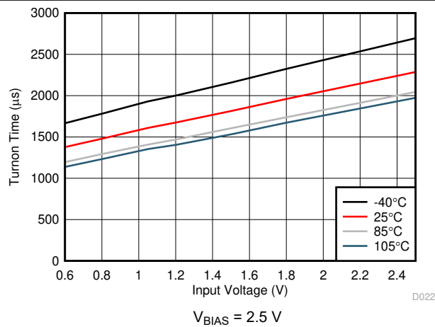
图 6-27. Turnon Time vs Input Voltage
