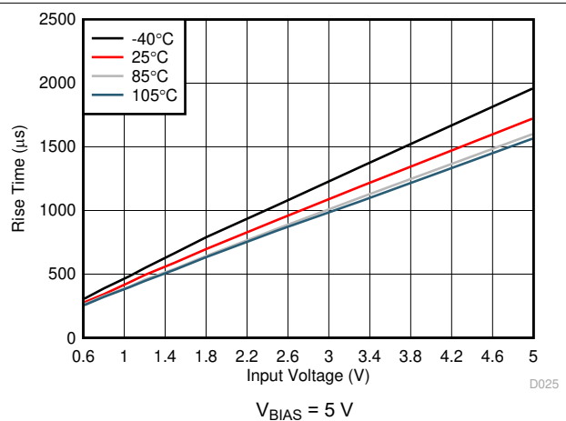
图 6-30. Rise Time vs Input Voltage
