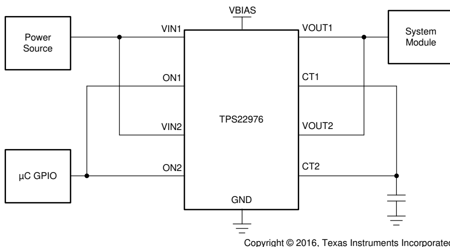
图 9-1. Parallel Configuration
