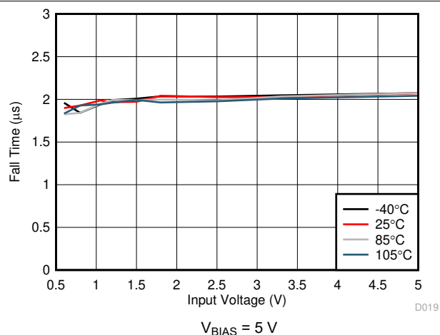
图 6-22. Fall Time vs Input Voltage
