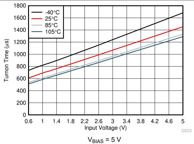
图 6-28. Turnon Time vs Input Voltage
