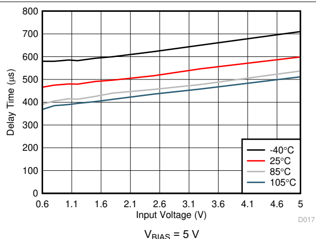
图 6-20. Delay Time vs Input Voltage
