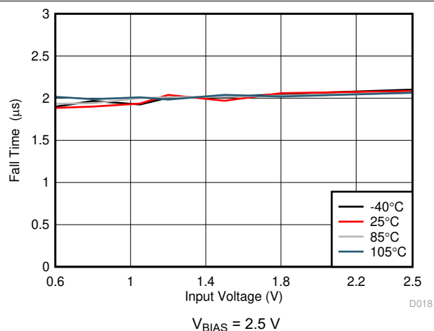
图 6-21. Fall Time vs Input Voltage
