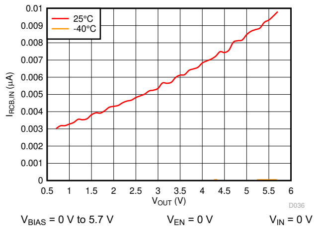
图 7-6. I_{RCB,IN} vs V_{OUT}
