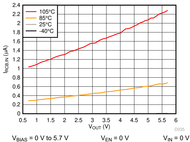
图 7-5. I_{RCB,IN} vs V_{OUT}
