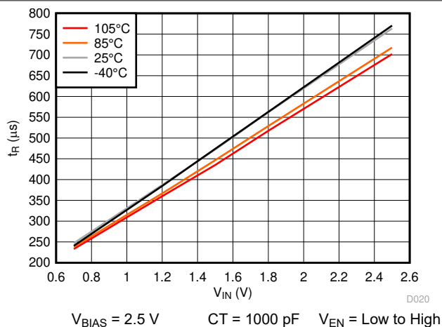
图 7-19. t_R vs V_{IN} , V_{BIAS} = 2.5 V
