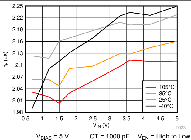
图 7-22. t_F vs V_{IN} , V_{BIAS} = 5 V
