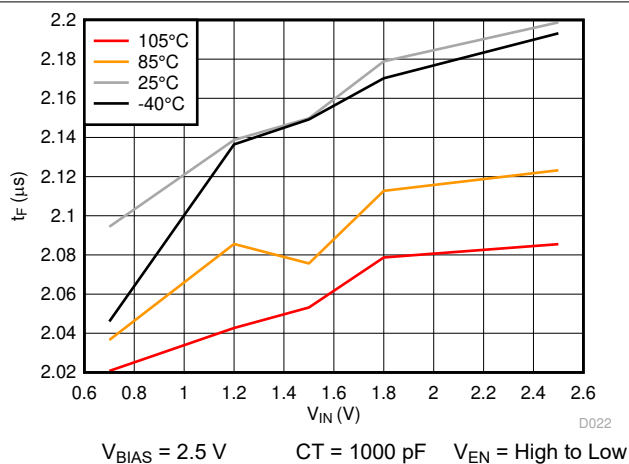
图 7-21. t_F vs V_{IN} , V_{BIAS} = 2.5 V
