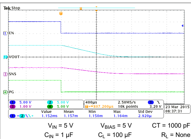
图 7-49. Quick Output Discharge of 100-µF Load ( t_{DIS} )
