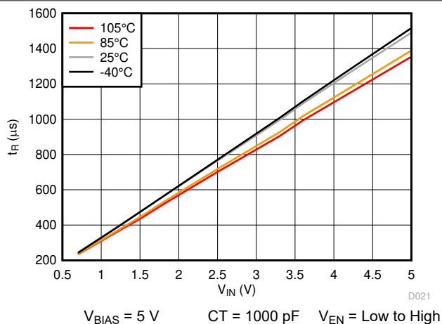
图 7-20. t_R vs V_{IN} , V_{BIAS} = 5 V
