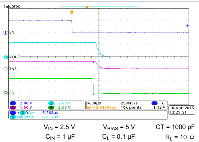
图 7-37. Turn-off Waveform, V_{BIAS} = 5 \text{ V}
