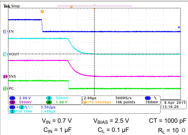
图 7-31. Turn-off Waveform, V_{BIAS} = 2.5\text{ V}
