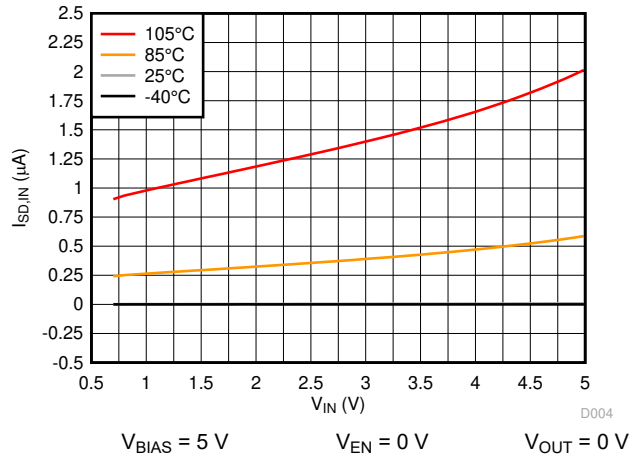
图 7-4. I_{SD,IN} vs V_{IN}
