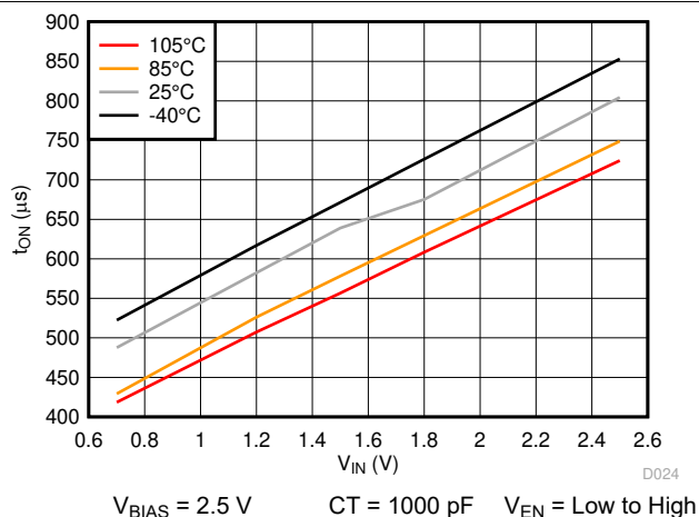
图 7-23. t_{ON} vs V_{IN} , V_{BIAS} = 2.5 V
