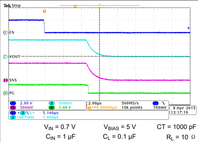
图 7-33. Turn-off Waveform, V_{BIAS} = 5\text{ V}
