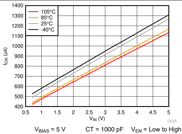
图 7-24. t_{ON} vs V_{IN} , V_{BIAS} = 5 V
