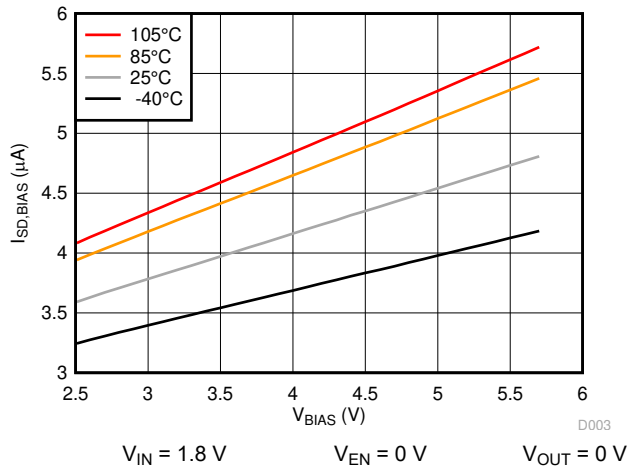
图 7-3. I_{SD,BIAS} vs V_{BIAS}
