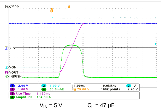
图 10-3. TPS22914C/15C Inrush Current
