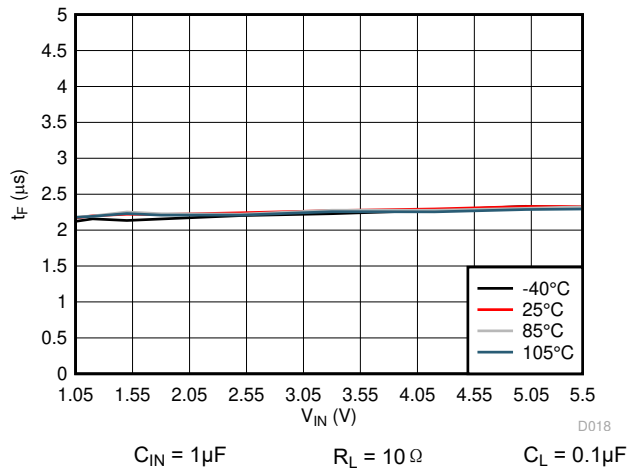
图 6-24. t_F 与 V_{IN} 间的关系
