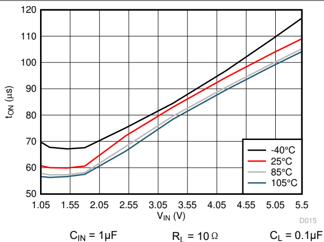
图 6-15. t_{ON} 与 V_{IN} 间的关系
