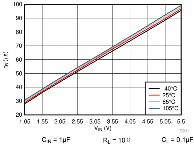
图 6-11. t_R 与 V_{IN} 间的关系
