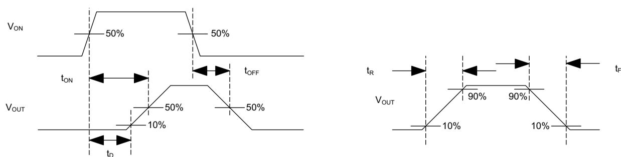
图 7-2. 时序波形
