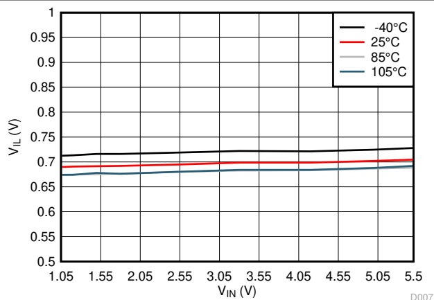
图 6-7. V_{IL} 与 V_{IN} 间的关系
