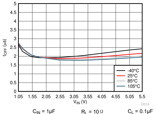
图 6-14. t_{OFF} 与 V_{IN} 间的关系
