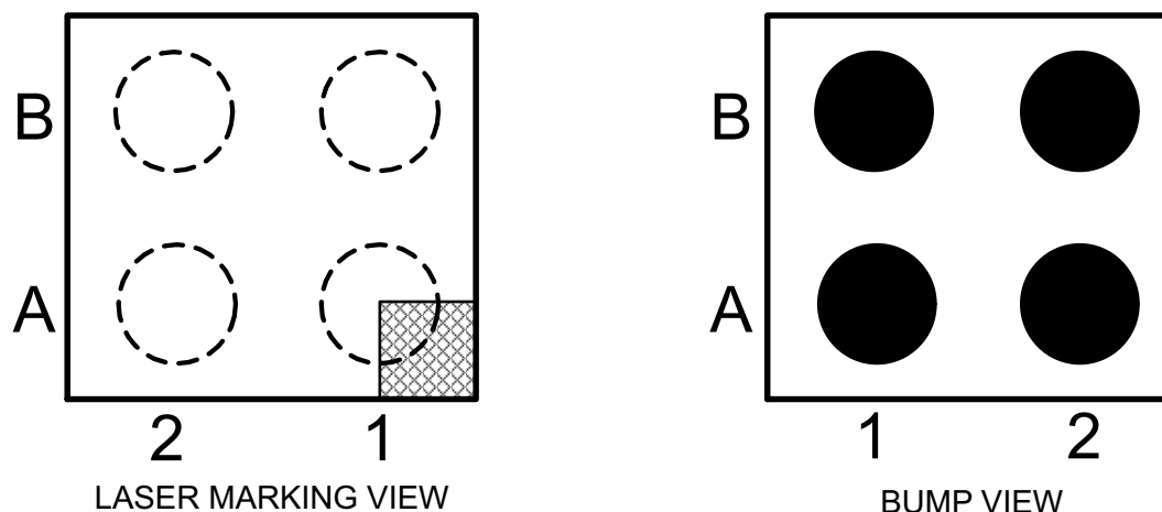
图 5-1. YFP 封装 4 引脚 DSBGA 顶视图
