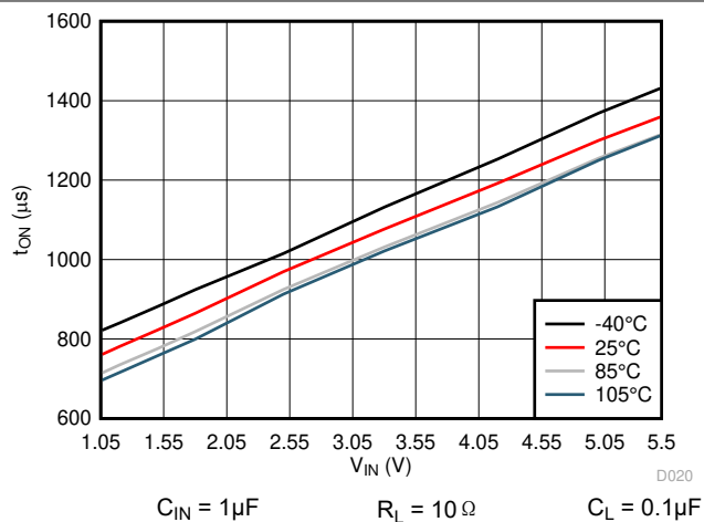
图 6-26. t_{ON} 与 V_{IN} 间的关系
