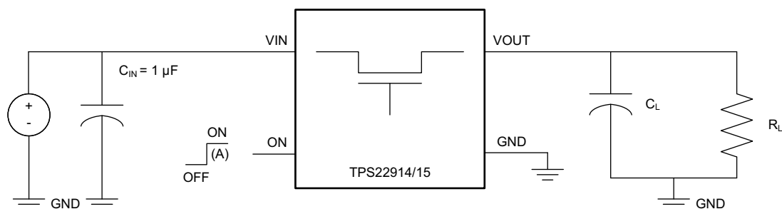
图 7-1. 测试电路
