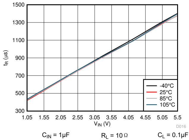
图 6-22. t_R 与 V_{IN} 间的关系
