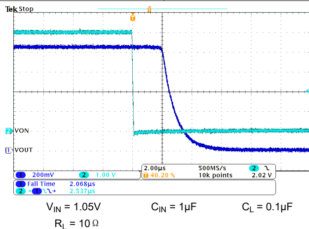
图 6-21. t_F = V_{IN} = 1.05V
