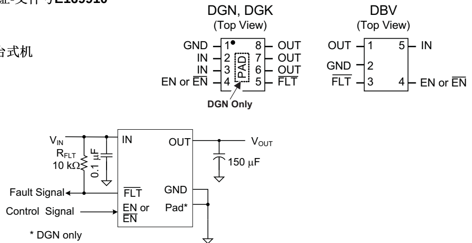
图 1. 典型应用
