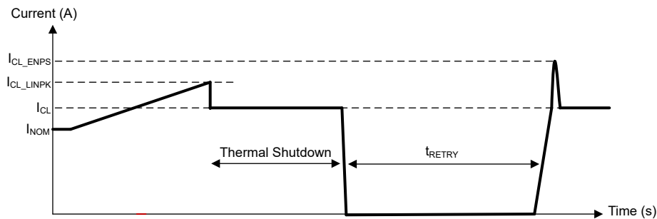
图 8-9. Overload Behavior
