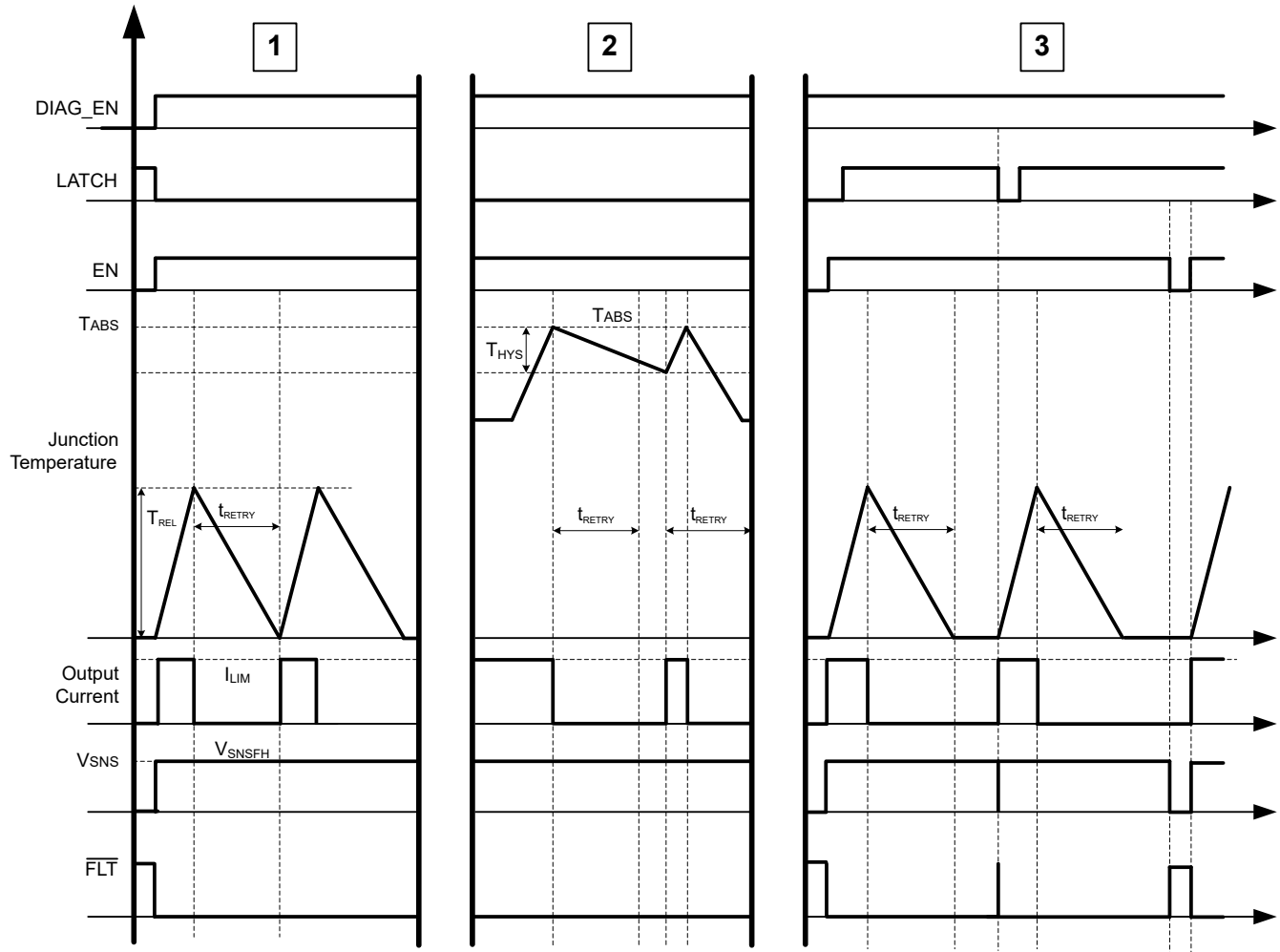
图 8-11. Thermal Behavior
