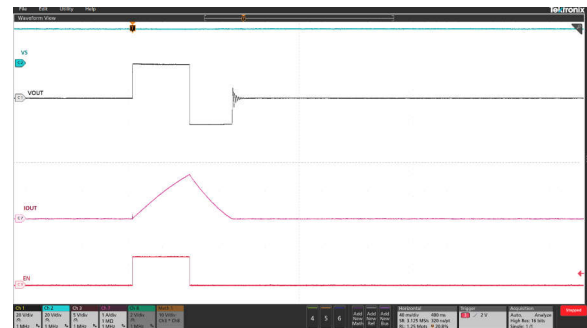
图 9-6. 400-mH Inductive Load Driving
