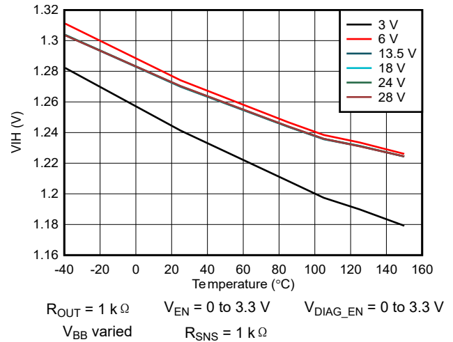
图 5-18. V_{IH} vs Temperature
