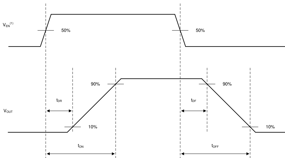
图 8-1. Parameter Definitions
