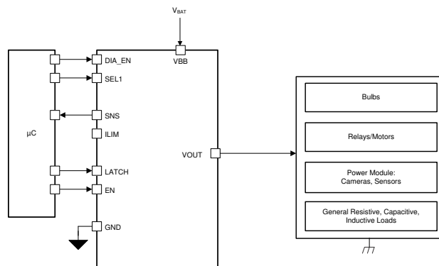
简化原理图
