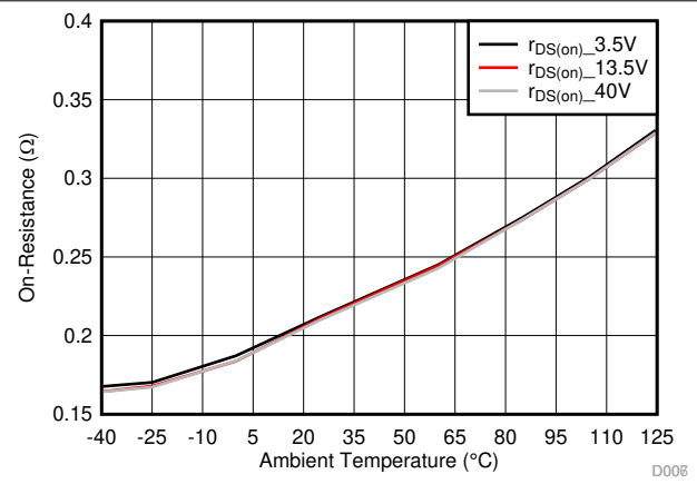
图 6-6. FET On-Resistance
