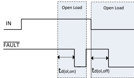
图 5-2. 负载开路消隐时间特性
