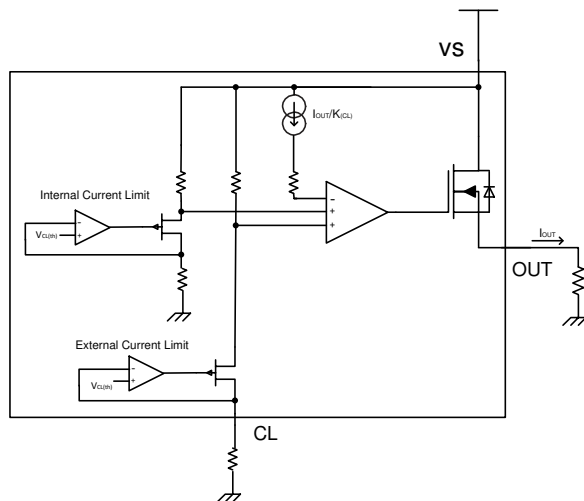
图 6-1. 电流限制
