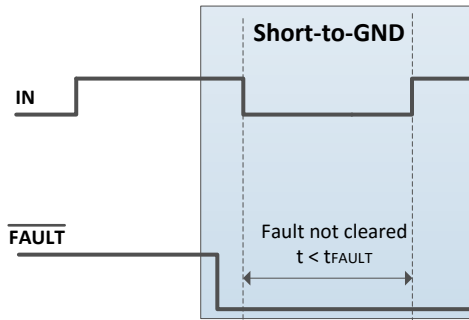
图 6-13. 具有故障报告保持功能
