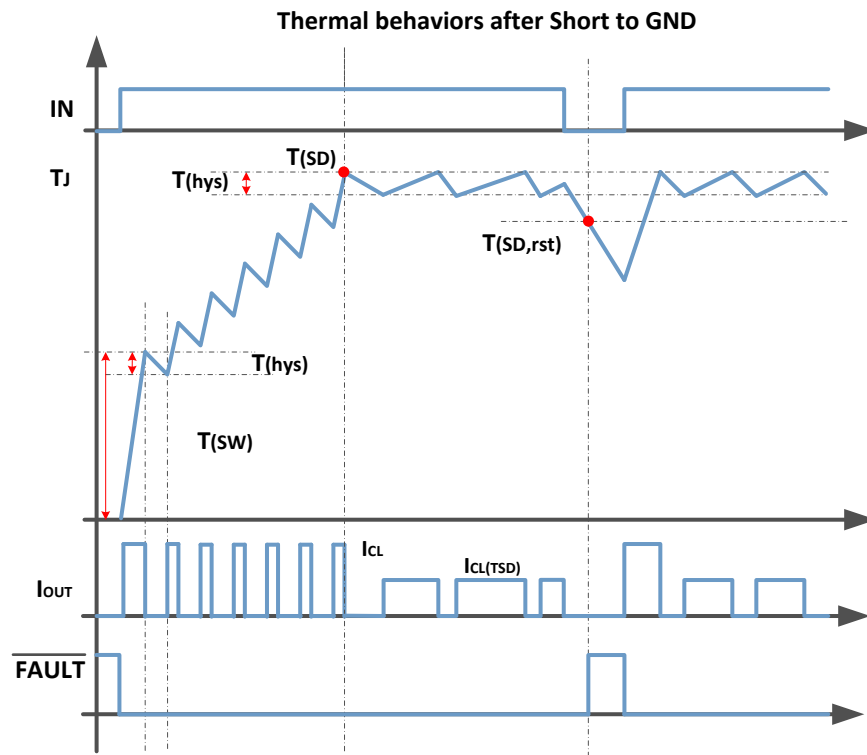
图 6-11. 热行为图
