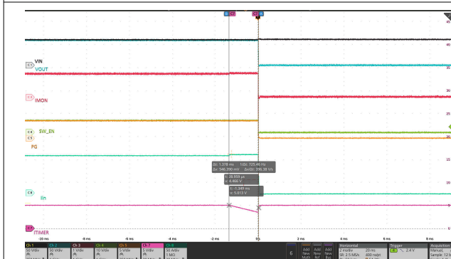
图 8-8. 断路器响应
