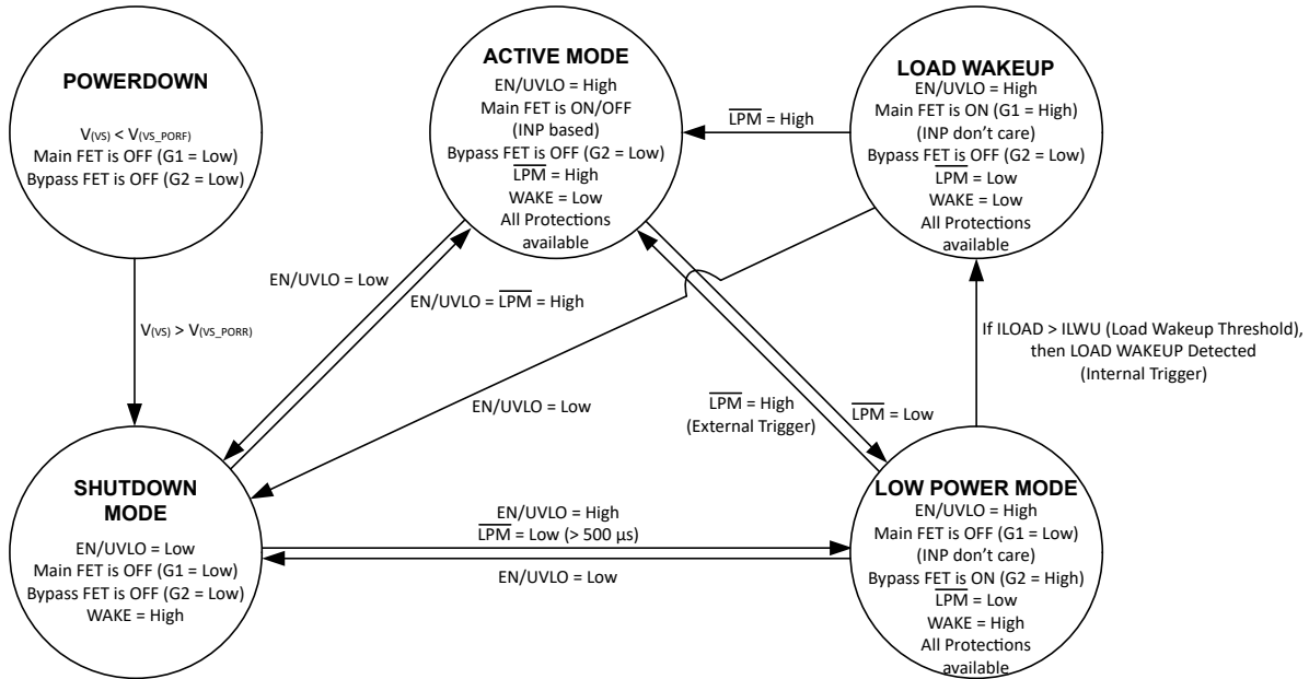
图 7-12. TPS12130-Q1 状态图
