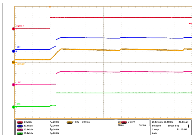
图 8-2. 低功耗路径的启动曲线 ( LPM = 低电平, V_{IN} = 12V , 无负载, CBST = 470nF )
