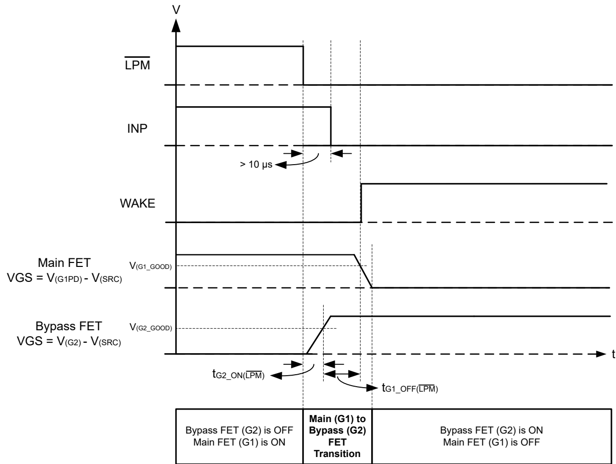
图 7-15. 从工作模式进入低功耗模式的 \overline{\text{LPM}} 和 \text{INP} 信号时序控制注意事项
