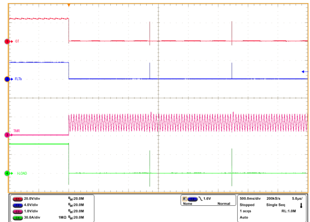
图 8-9. TPS12130-Q1 针对过流故障的自动重试响应
