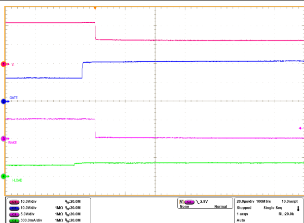
图 9-4. 从 LPM 到工作模式的状态转换放大视图 ( \overline{\text{LPM}} = 低电平, V_{\text{IN}} = 12\text{V} , \text{EN/UVLO} = 高电平)
