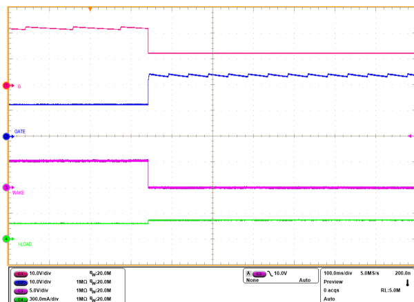
图 9-3. 从 LPM 到工作模式的状态转换 ( \overline{\text{LPM}} = 低电平, V_{\text{IN}} = 12\text{V} , \text{EN/UVLO} = 高电平)
