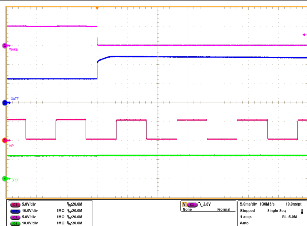
图 9-5. 当负载唤醒状态下 \overline{\text{LPM}} = 低电平时, \text{INP} 无法控制 \text{GATE}
