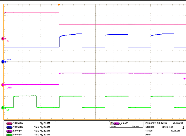
图 9-7. 当 \overline{\text{LPM}} = 低电平到高电平时, \text{INP} 获得对 \text{GATE} 的控制 ( V_{\text{IN}} = 12\text{V} , 无负载)
