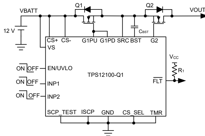
图 8-11. 简单栅极驱动器的 TPS12100-Q1 应用电路
