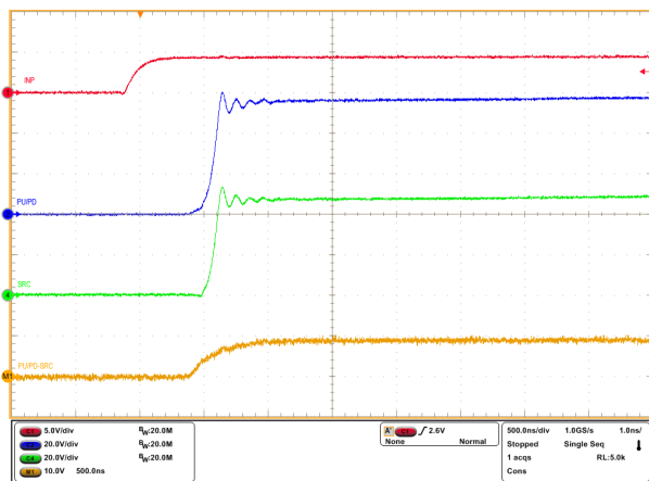
图 9-4. INP1 由低电平到高电平且 C_{BST} = 470nF 时 TPS12100-Q1 的导通响应
