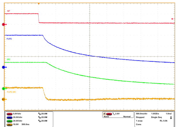
图 9-5. INP1 由高电平到低电平且 C_{BST} = 470nF 时 TPS12100-Q1 的关断响应
