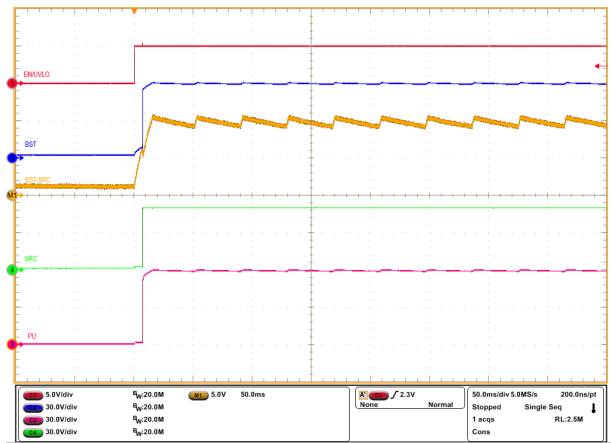
图 9-3. INP1=INP2 = HIGH 且 C_{BST} = 470nF 时自举电压的启动曲线
