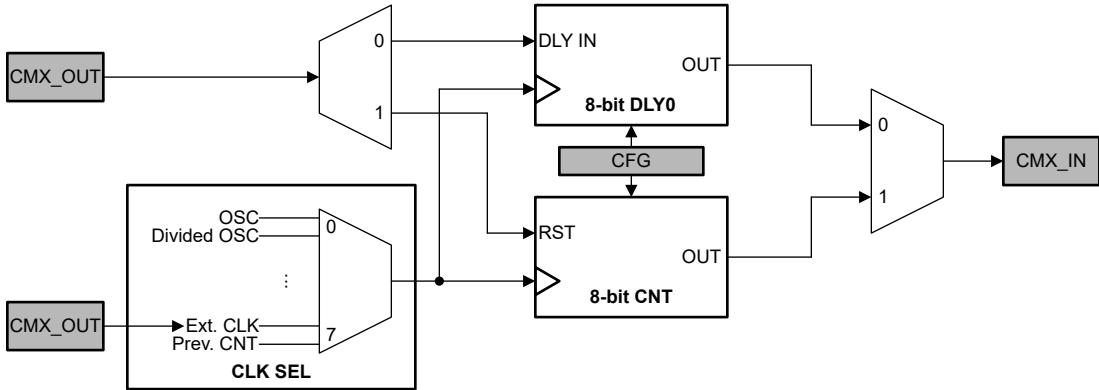
图 7-9. CNT/DLY 方框图
