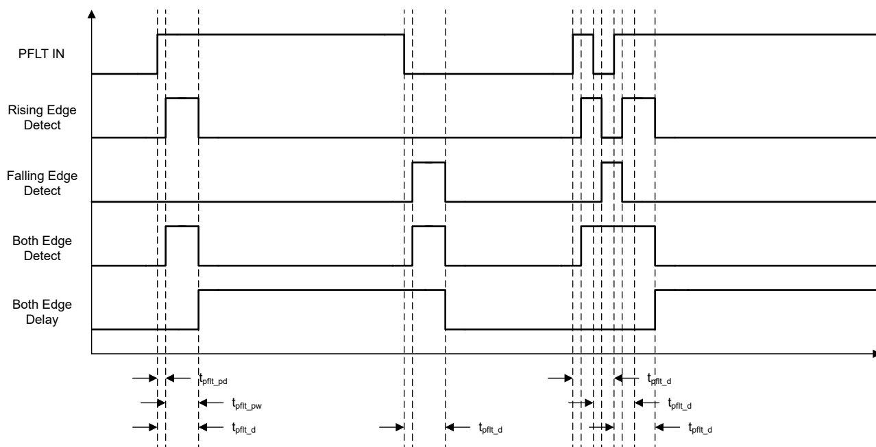
图 7-17. 可编程滤波器和边沿检测器输出时序图示例
