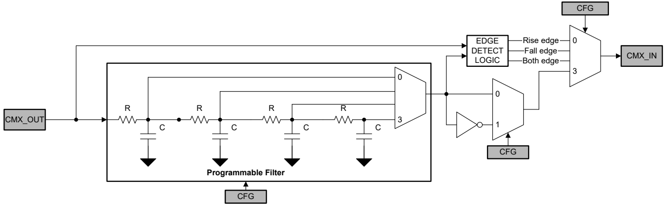
图 7-17. 可编程滤波器和边沿检测器方框图
