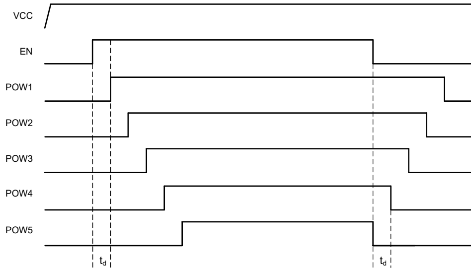
图 8-2. 应用时序图
