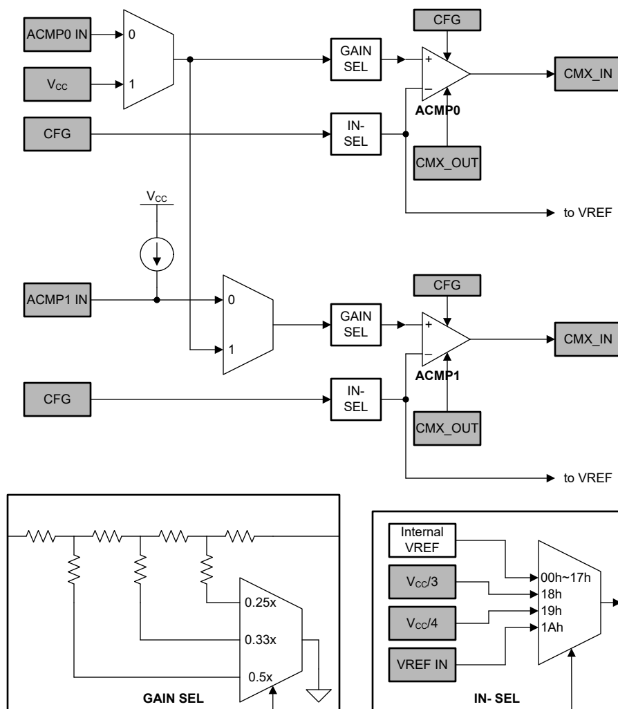
图 7-20. ACMP 方框图
