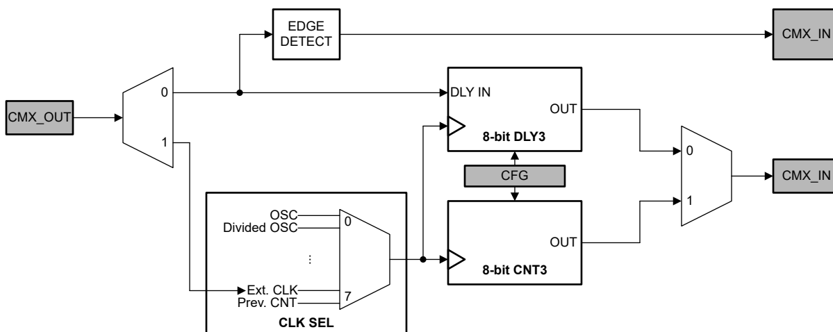
图 7-10. CNT/DLY3 方框图
