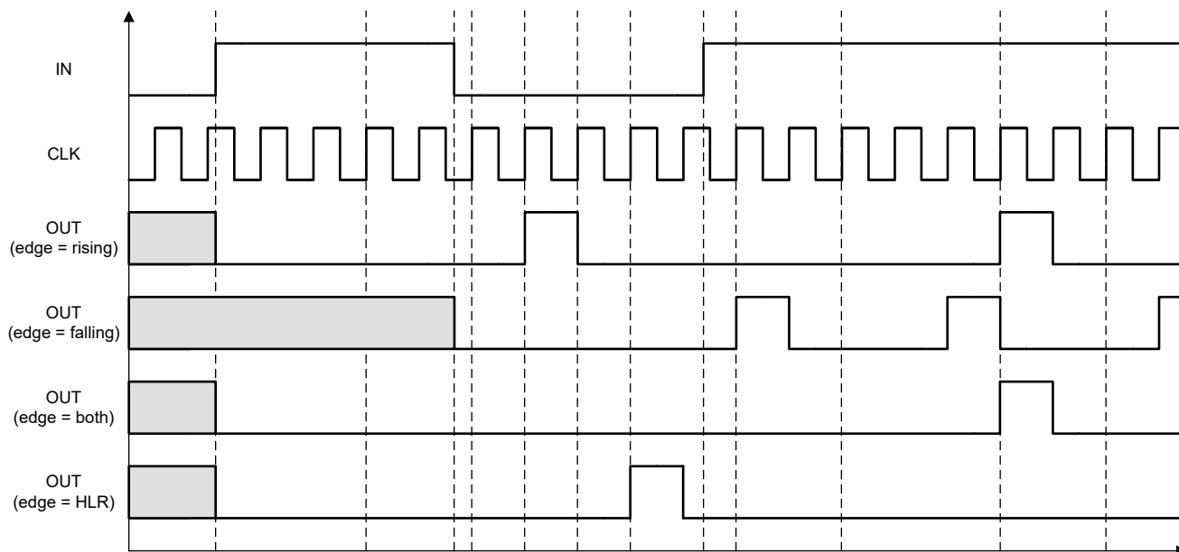
图 7-16. RST &lt; DATA (DATA = 3) 的计数器输出时序示例
