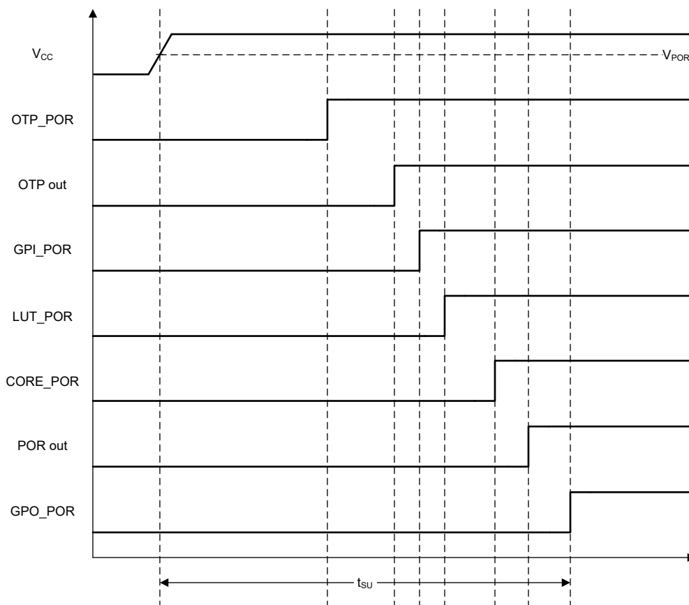
图 7-22. POR 序列
