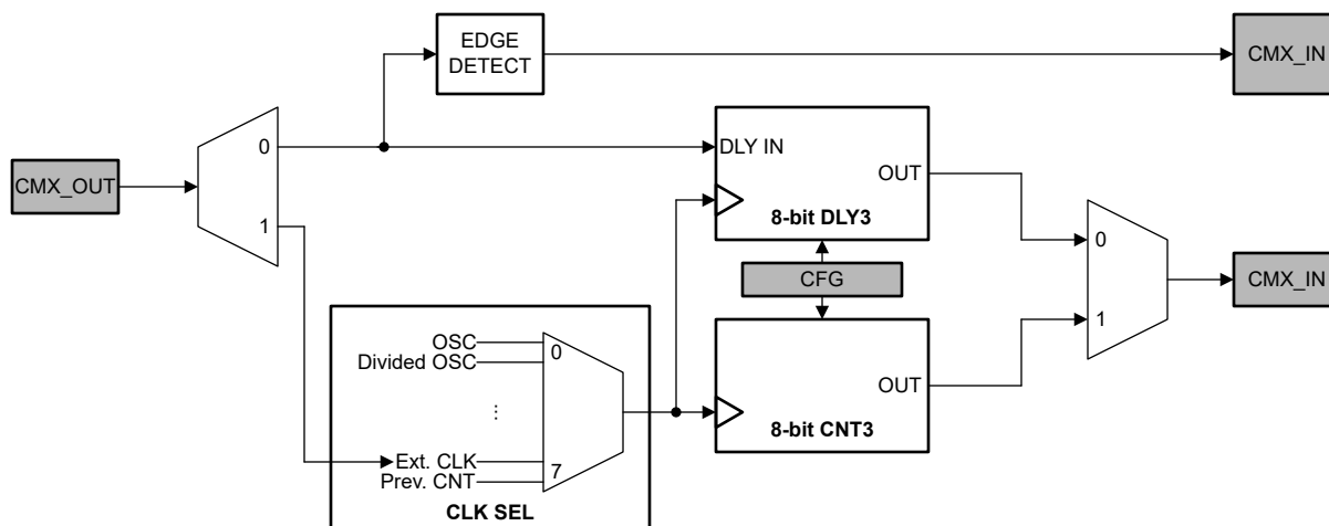
图 7-10. CNT/DLY3 方框图
