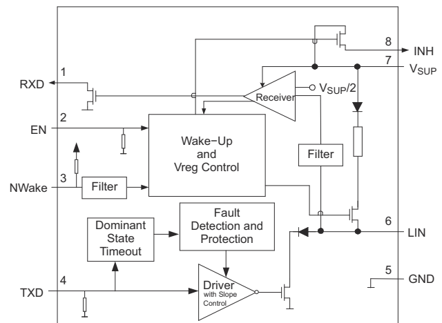
功能方框图
