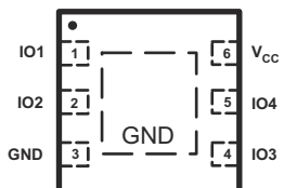
图 4-3. DRS 封装 6 引脚 SON 顶视图
