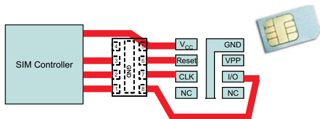
图 1. 在 SIM 卡接口上使用 TPD3F303 的电路板布局
