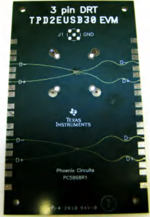
图 10-3. TPDxUSB30/A EVM - TPD2EUSB30/A Side
