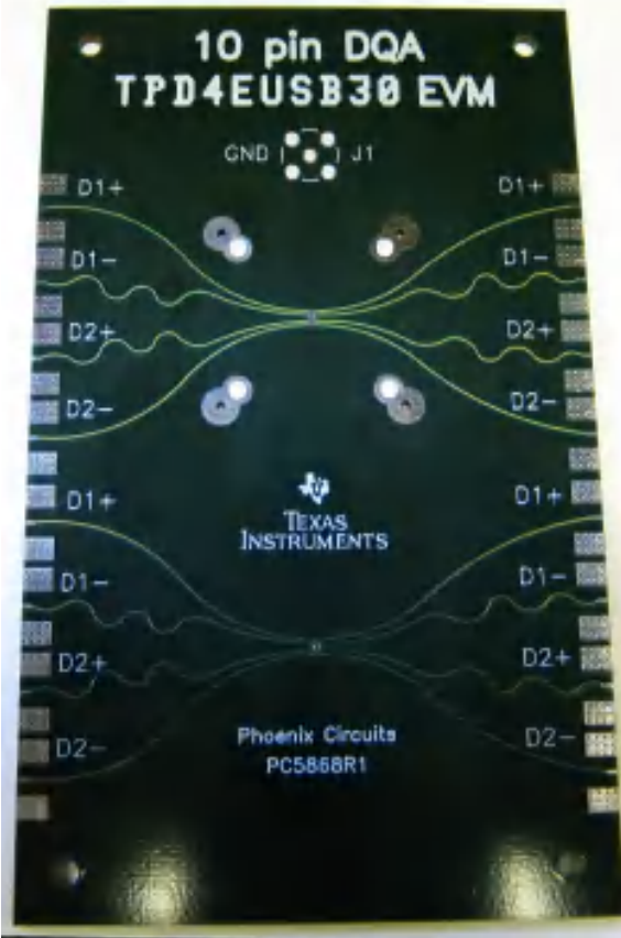
图 10-2. TPDxUSB30/A EVM - TPD4EUSB30 Side
