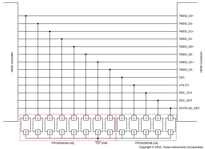
典型的 HDMI 2.0 应用
